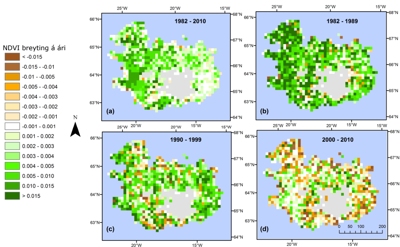
Mynd 8.5 Leitni í hámarksgróðurstuðli (NDVI) á Íslandi að sumri eftir tímabilum á árunum 1982–2010. Vesturland og Norðvesturland eru meðal svæða þar sem grænkun varð hvað mest á tímabilinu. (Heimild: sjá tilvísun 33.)
