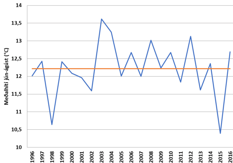
Mynd 8.14 Meðalhiti júní – ágúst í Laxá í Aðaldal mældur með sírita við Laxamýri.
