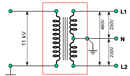
Mynd 6.20 Tvífasa rafkerfi 2/N~460/230 V
