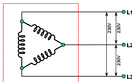
Mynd 6.19 Þrífasa rafkerfi 3/230 V
