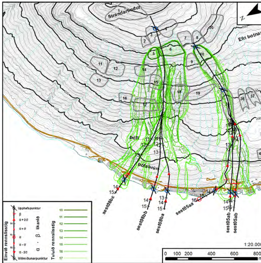
Mynd 19. Niðurstöður SamosAT líkanreikninga fyrir upptakasvæði 5, 6 og 10.
