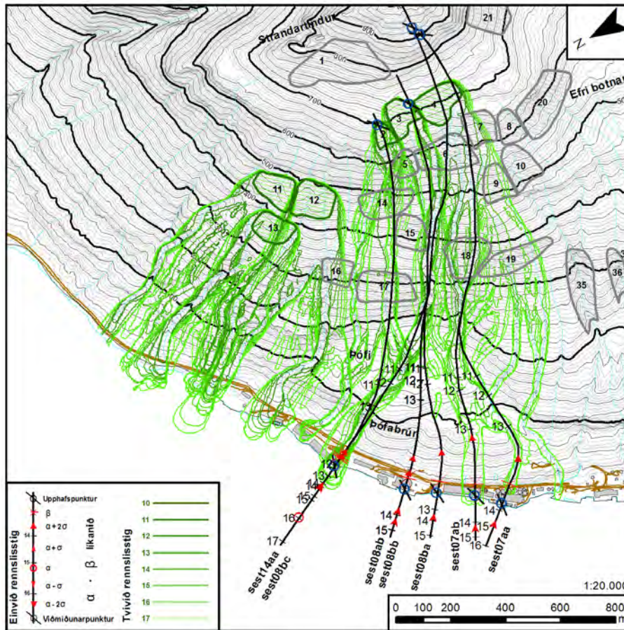
Mynd 18. Niðurstöður SamosAT líkanreikninga fyrir upptakasvæði 2–4, 8 og 11–13.
