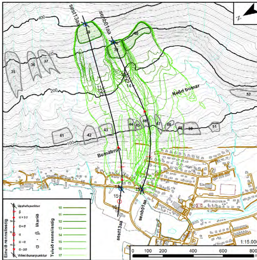
Mynd 27. Niðurstöður SamosAT líkanreikninga fyrir upptakasvæði 38–40 ofan Neðri-Botna.
