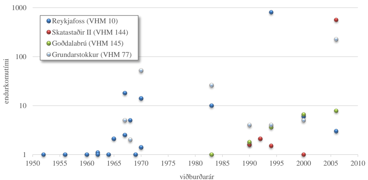
Mynd III-13. Endurkomutími rennslis skráðra flóðaatburða við Reykjafoss (VHM 10), Grundarstokk (VHM 77), Skatastaði (VHM 144) og Goðdalabrá (VHM 145).
