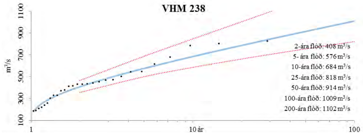
Mynd VI-3. Niðurstöður tíðnigreiningar fyrir VHM 238. Línuritið sýnir reiknuð og mæld hæstu flóð ásamt 95% vikmörkum (brotin, rauð lína).
