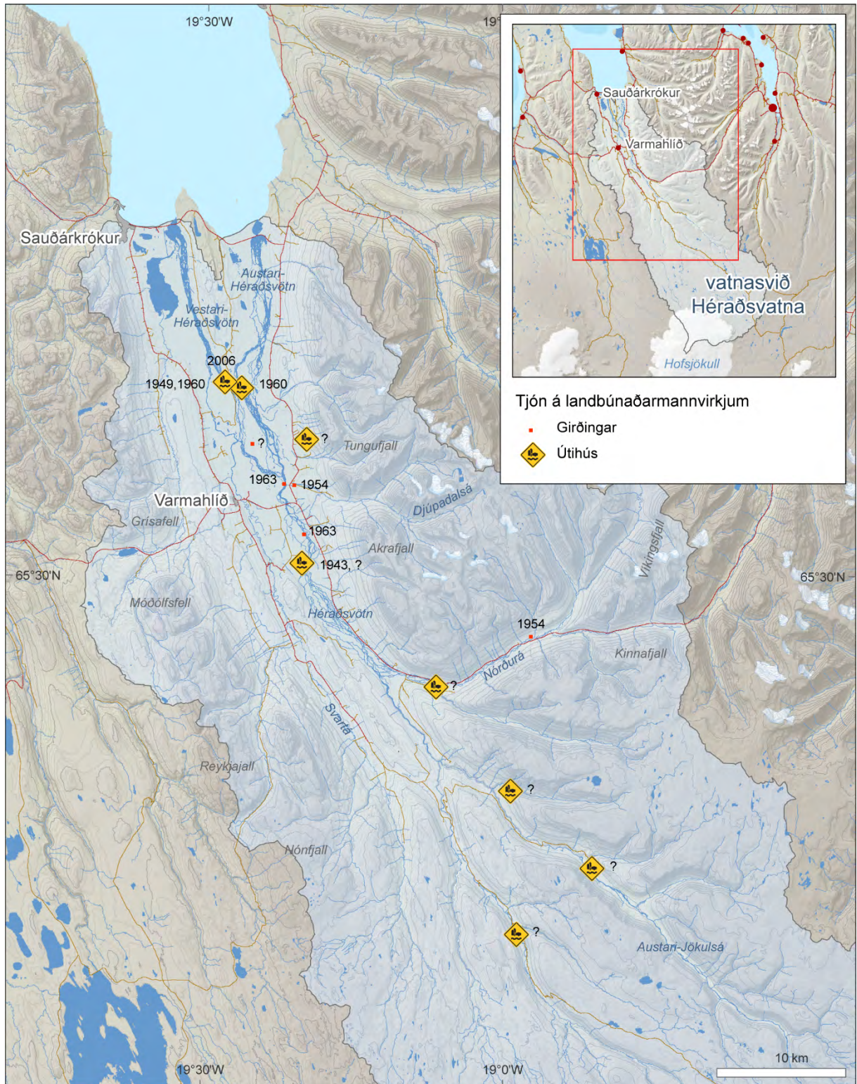
Mynd III-21. Tjón á landbúnaðarmannvirkjum af völdum flóða á vatnasviði Héraðsvatna.
