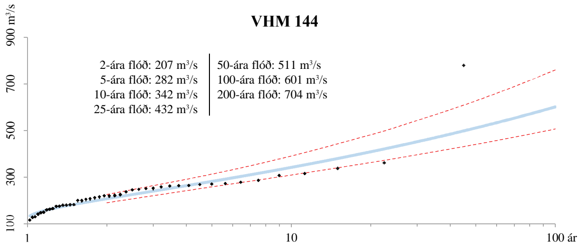
Mynd III-3. Niðurstöður tíðnigreiningar fyrir VHM 144 í Austari-Jökulsá. Línuritið sýnir reiknuð og mæld hæstu flóð ásamt 95% vikmörkum (brotin lína).
