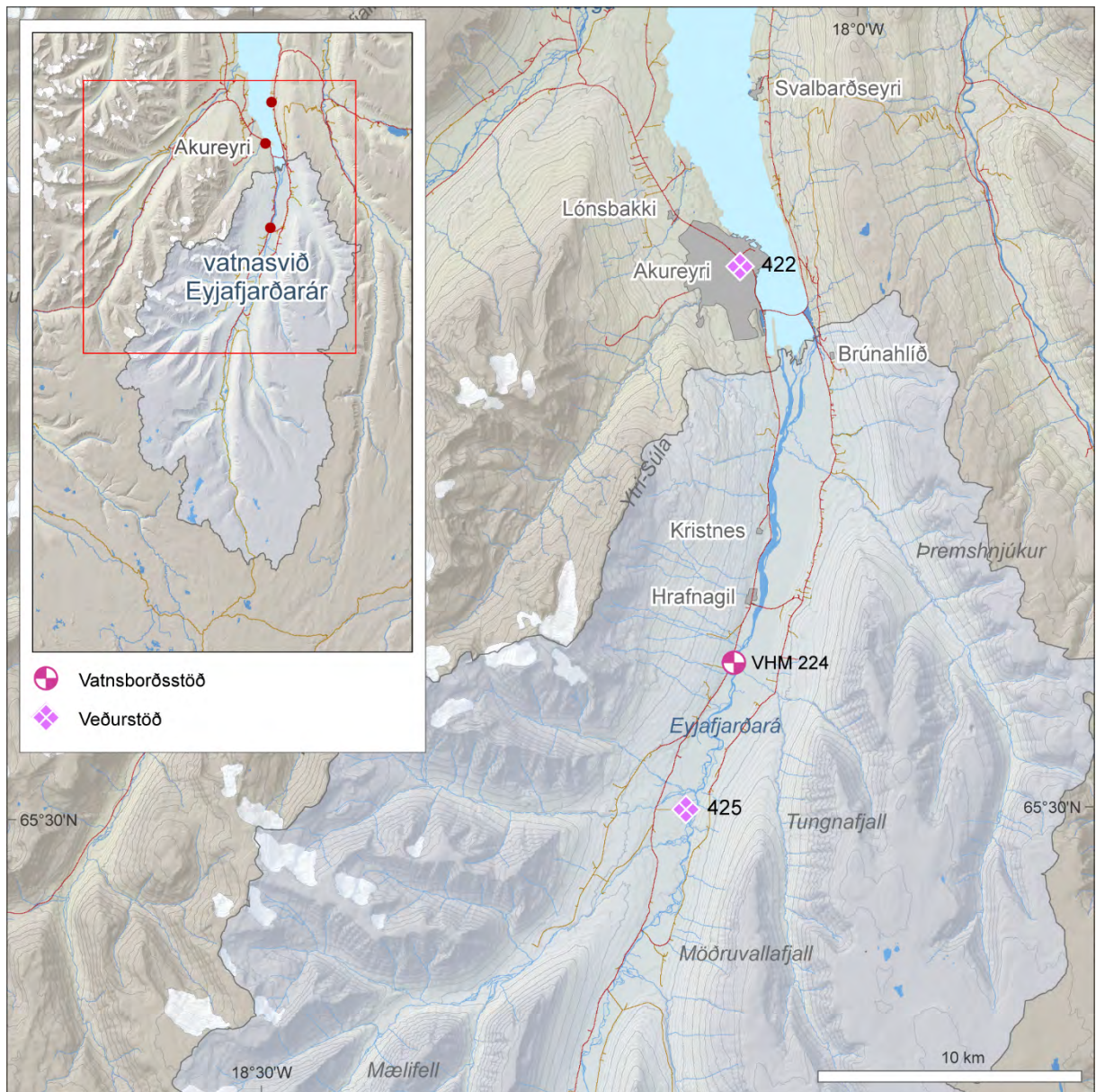
Mynd II-2. Staðsetning veður- og vatnsborðsstöðva sem notaðar voru til að greina flóð á vatnasviði Eyjafjarðarar.
