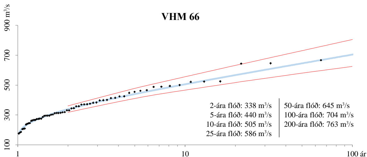
Mynd IV-3. Niðurstöður tíðnigreiningar fyrir VHM 66. Línuritíð sýnir reiknuð og mæld hæstu flóð ásamt 95% vikiörkum (brotin lína).
