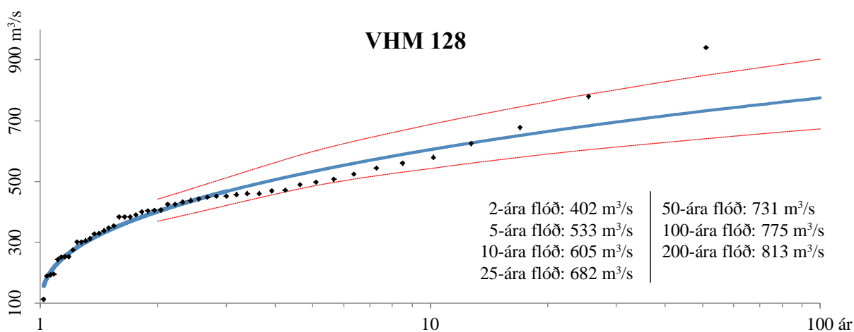
Mynd IV-4. Niðurstöður tíðnigreiningar fyrir VHM 128. Línuritíð sýnir reiknuð og mæld hæstu flóð ásamt 95% vikiörkum (brotin lína).
