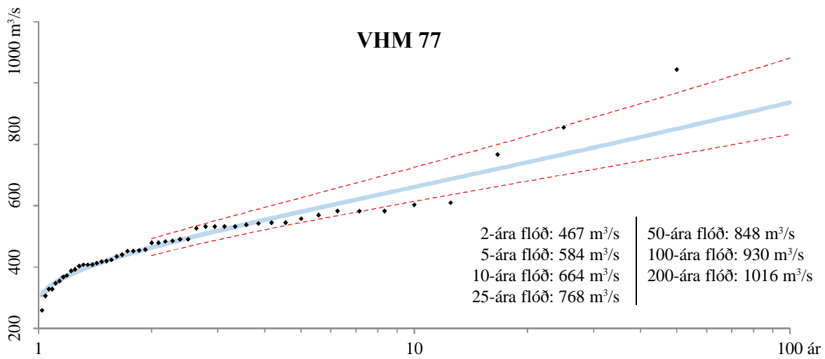
Mynd III-5. Niðurstöður tíðnigreiningar fyrir VHM 77 í Héraðsvötnum. Línuritið sýnir reiknuð og mæld hæstu flóð ásamt 95% vikiörkum (brotin lína).
