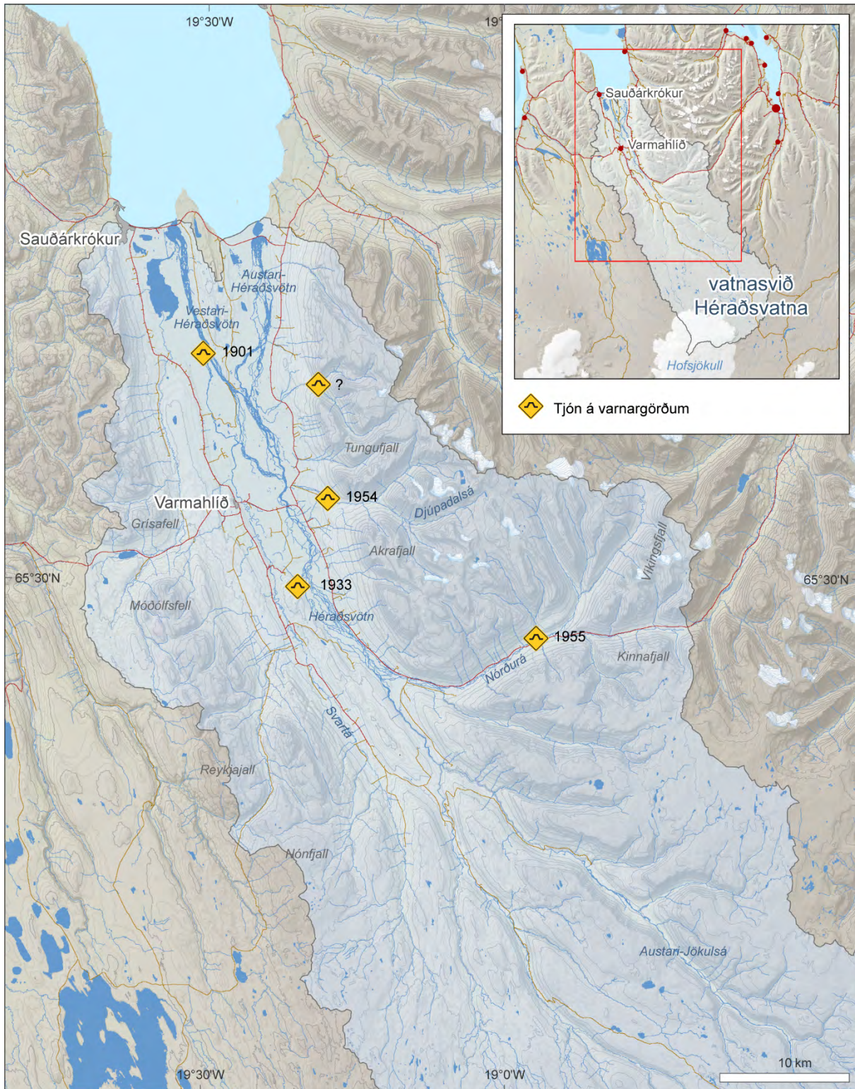
Mynd III-20. Tjón á varnargörðum af völdum flóða á vatnasviði Héraðsvatna.
