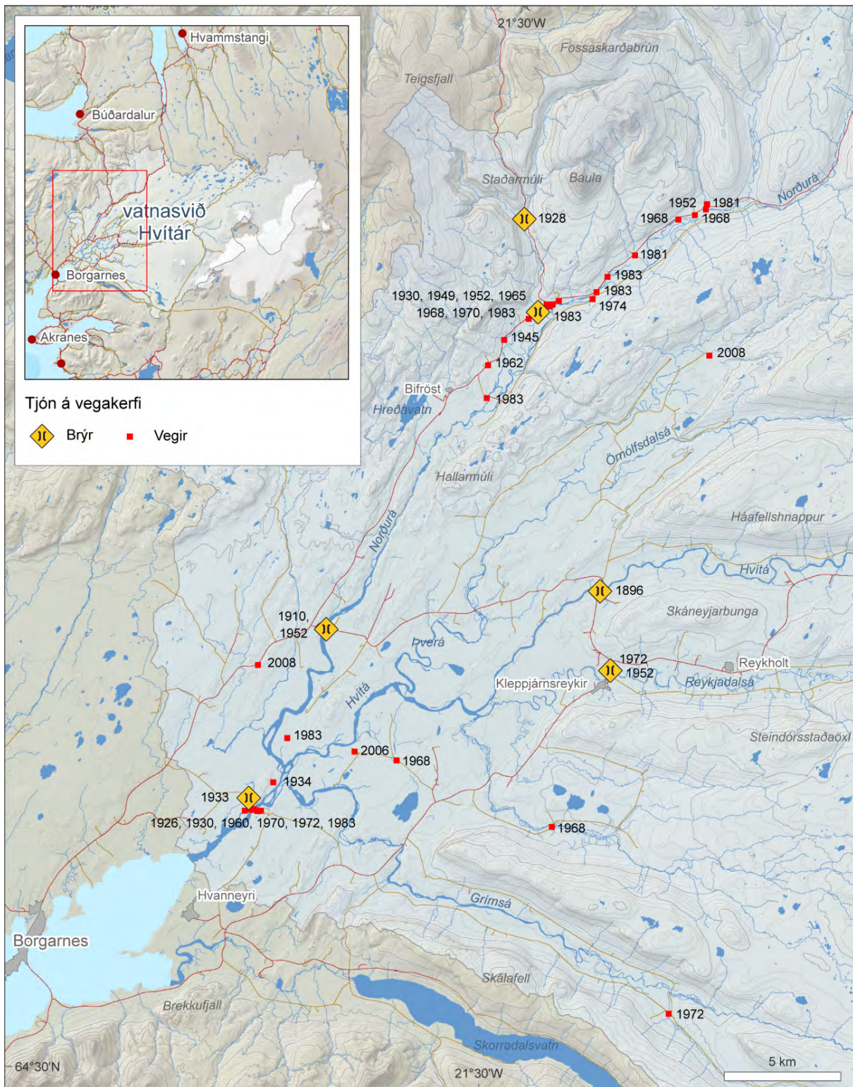
Mynd IV-12. Tjón á vegakerfi af völdum flóða á vatnasviði Hvítár.
