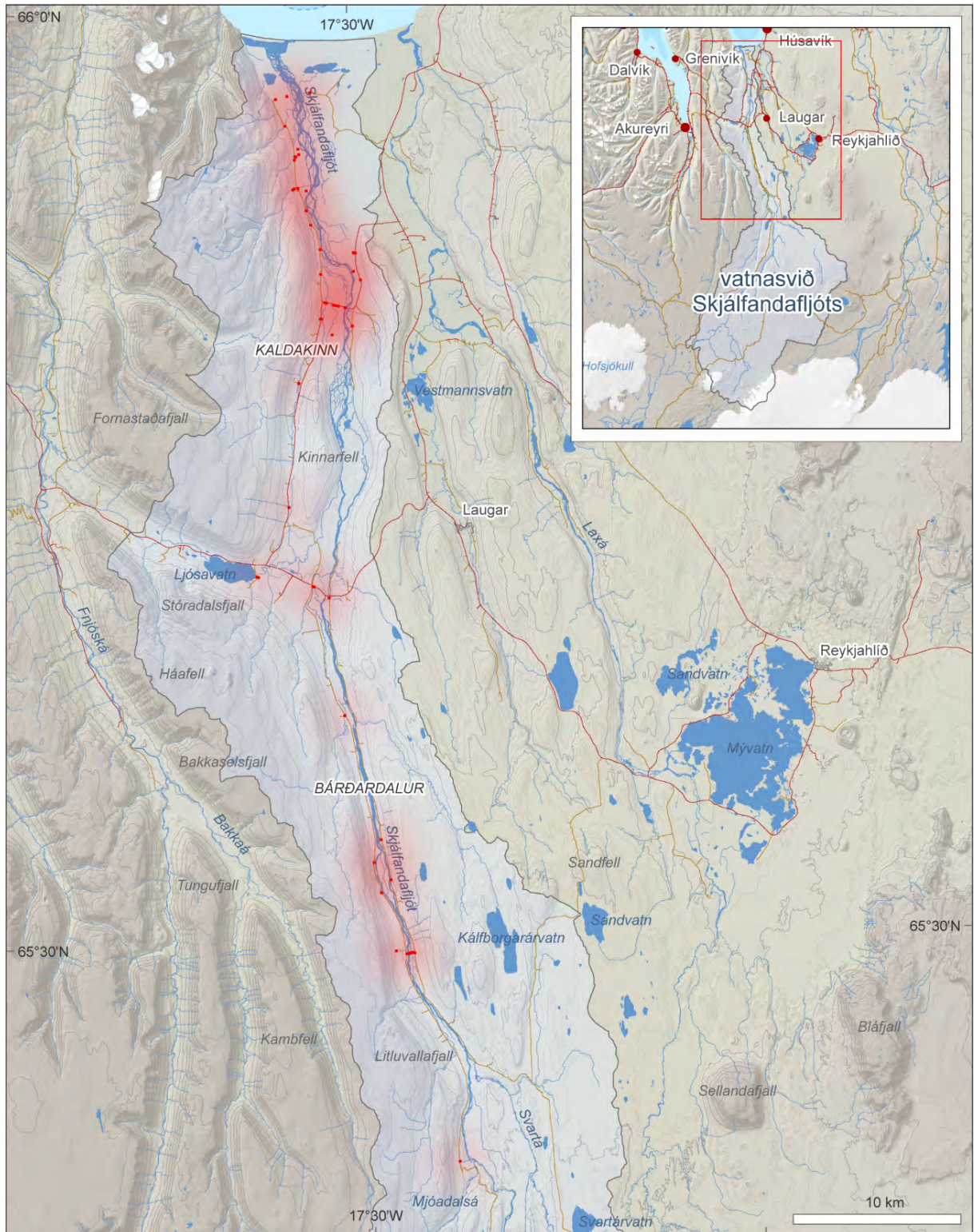
Mynd VI-9. Tjónspor (rauð móða) vatnsflóða á vatnasviði Skjálfandafhljóts samkvæmt staðsetningu tjóna á samgöngukerfinu og íbúðarhúsum.
