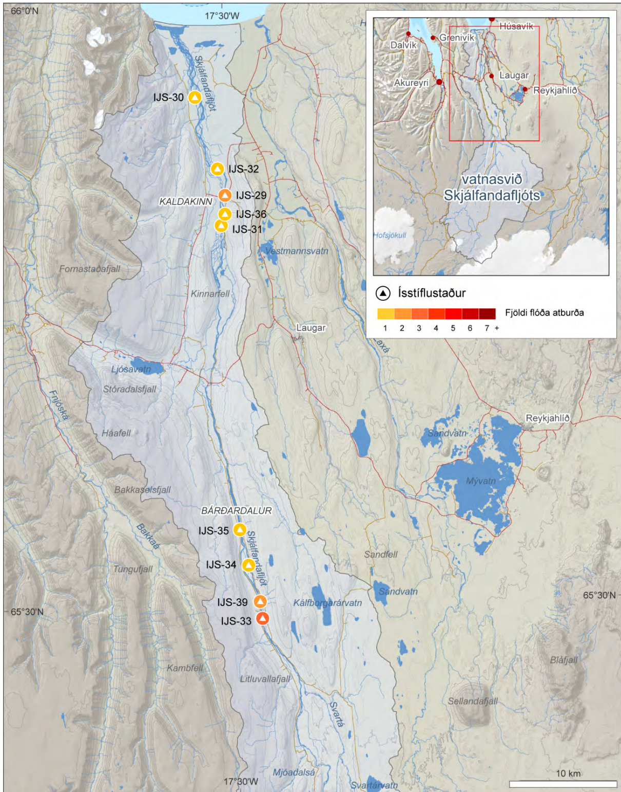
Mynd VI-6. Greindir ísstíflustaðir á vatnasviði Skjálfandafhljóts.
