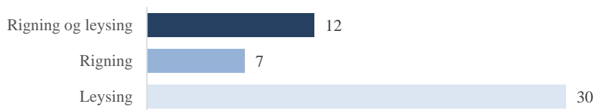
Mynd III-9. Veðurorsakir flóða í Héraðsvötnum.
