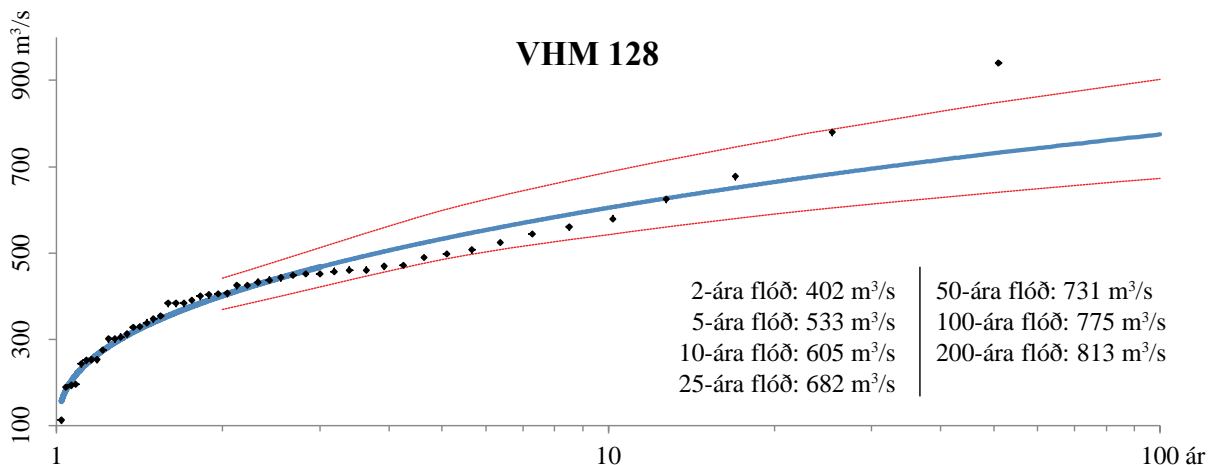
Mynd I-2. Niðurstöður tíðnigreiningar fyrir VHM128. Línuritið sýnir reiknuð og mæld hæstu flóð ásamt 95% vikmörkum (brotin lína).
