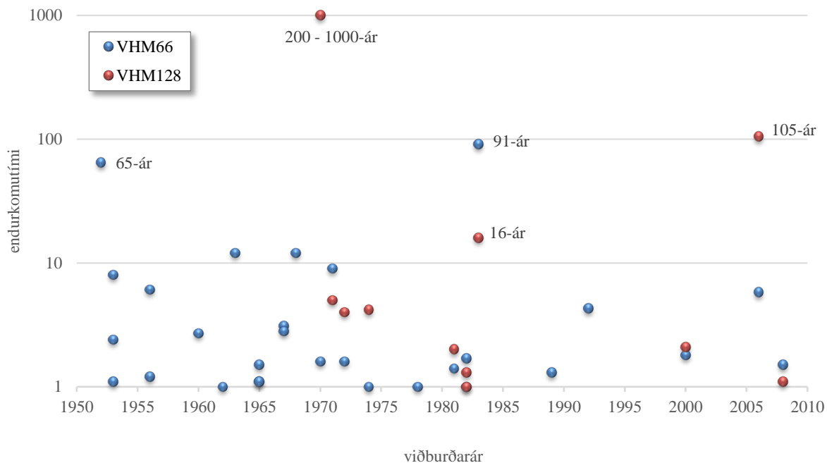
Mynd IV-10. Endurkomutími rennslis skráðra flóðaatburða við Kljáfoss (VHM 66) og Stekk (VHM 128).
