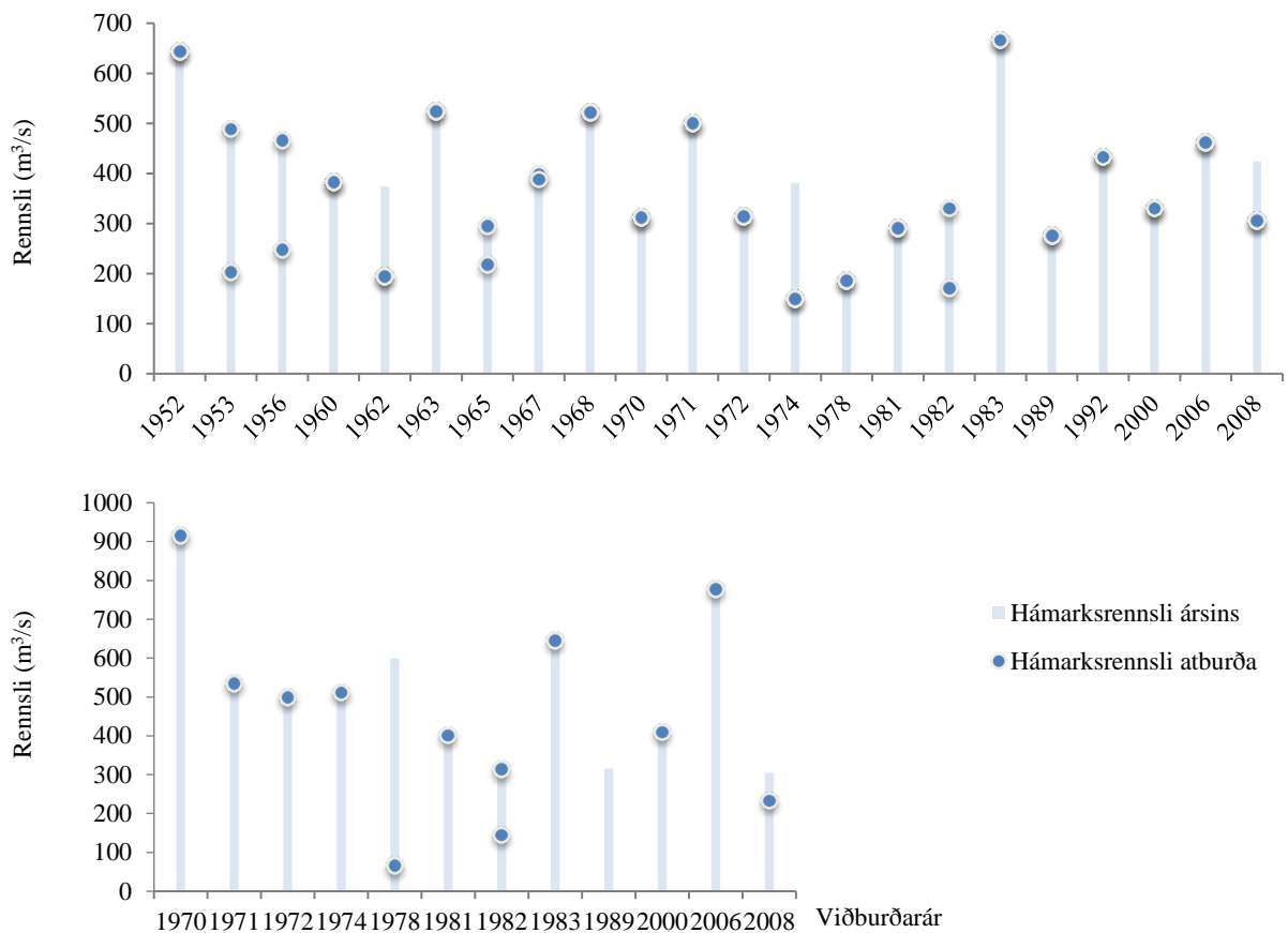
Mynd IV-9. Samanburður milli rennslis skráðra atburða og mesta rennslis ársins við Kljáfoss annars vegar (efri mynd) og Stekk hins vegar (neðri mynd).
