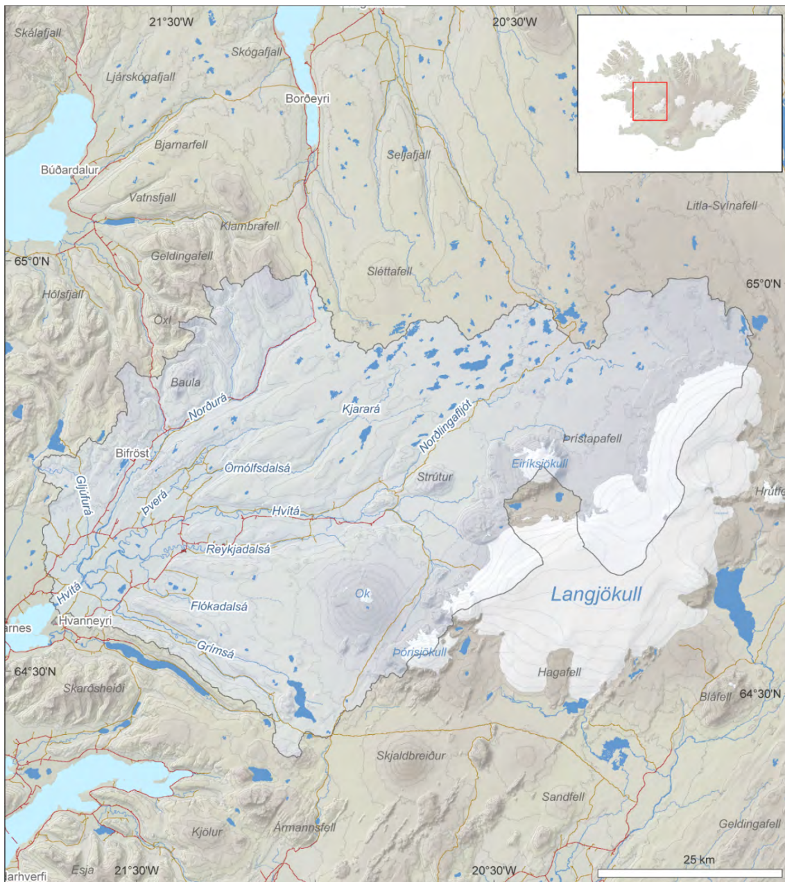
Mynd IV-1. Vatnasvið Hvítár í Borgarfirði (blátt svæði) og helstu ár innan vatnasviðsins.
