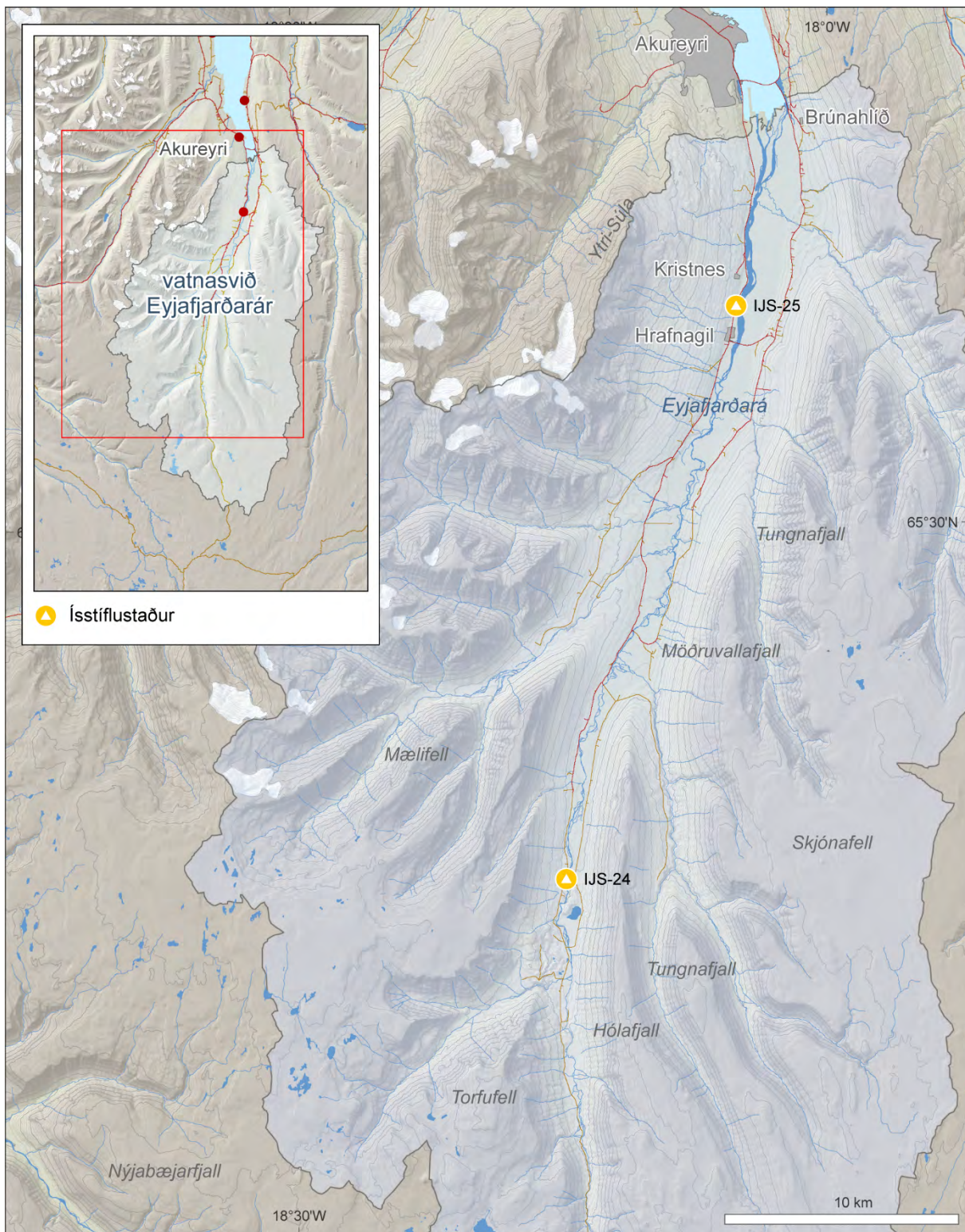
Mynd II-6. Greindir ísstíflustaðir á vatnasviði Eyjafjarðarár.
