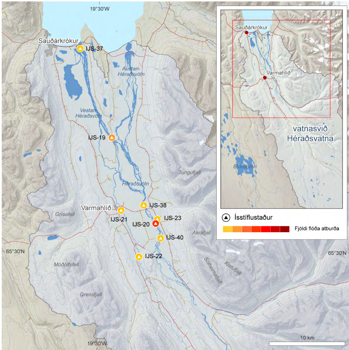
Mynd III-11. Greindir ísstíflustaðir á vatnasviði Héraðsvatna.
