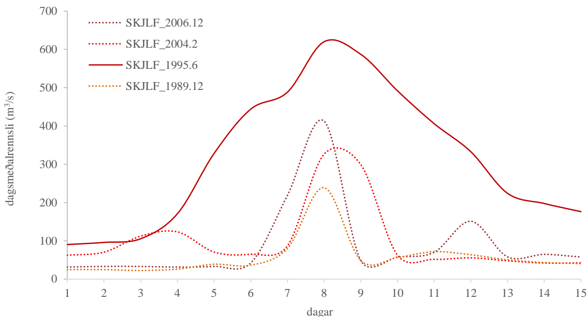
Mynd VI-7. Breytingar í dagsmeðalrennslis atburðanna 1989, 1995, 2004 og 2006.
