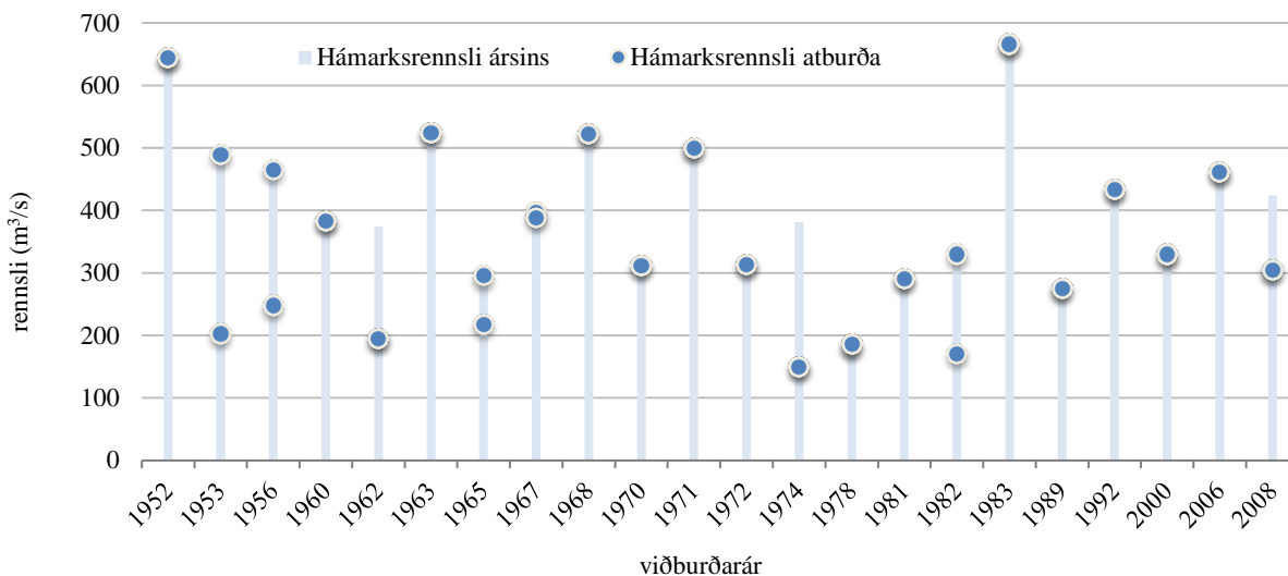
Mynd I-3. Samanburður milli rennslis skráðra atburða og mesta rennslis ársins við Kljáfoss (VHM 66). Flóð sem eru skráð í gagnabanka sögulegra flóða vegna þess tjóns og þeirrar röskunar sem þau ollu, þurfa ekki endilega að hafa verið stærstu flóð ársins sem koma fram við viðkomandi vatnshæðarmæli.
