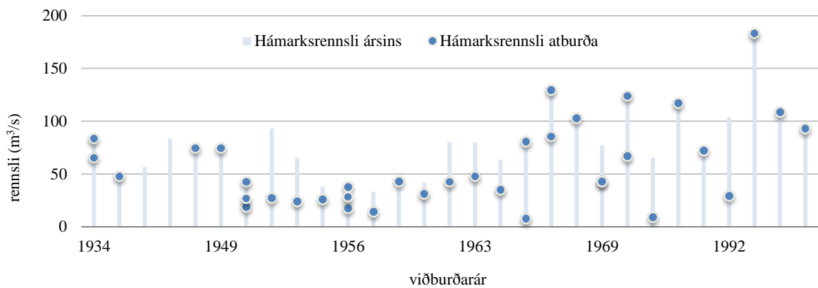
Mynd III-12. Samanburður milli rennslis skráðra atburða og mesta rennslis ársins, við Svartá (VHM 10).
