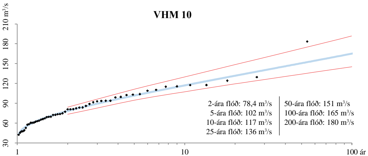
Mynd III-6. Niðurstöður tíðnigreiningar fyrir VHM 10 í Svartá. Línuritið sýnir reiknuð og mæld hæstu flóð ásamt 95% vikiörkum (brotin lína).
