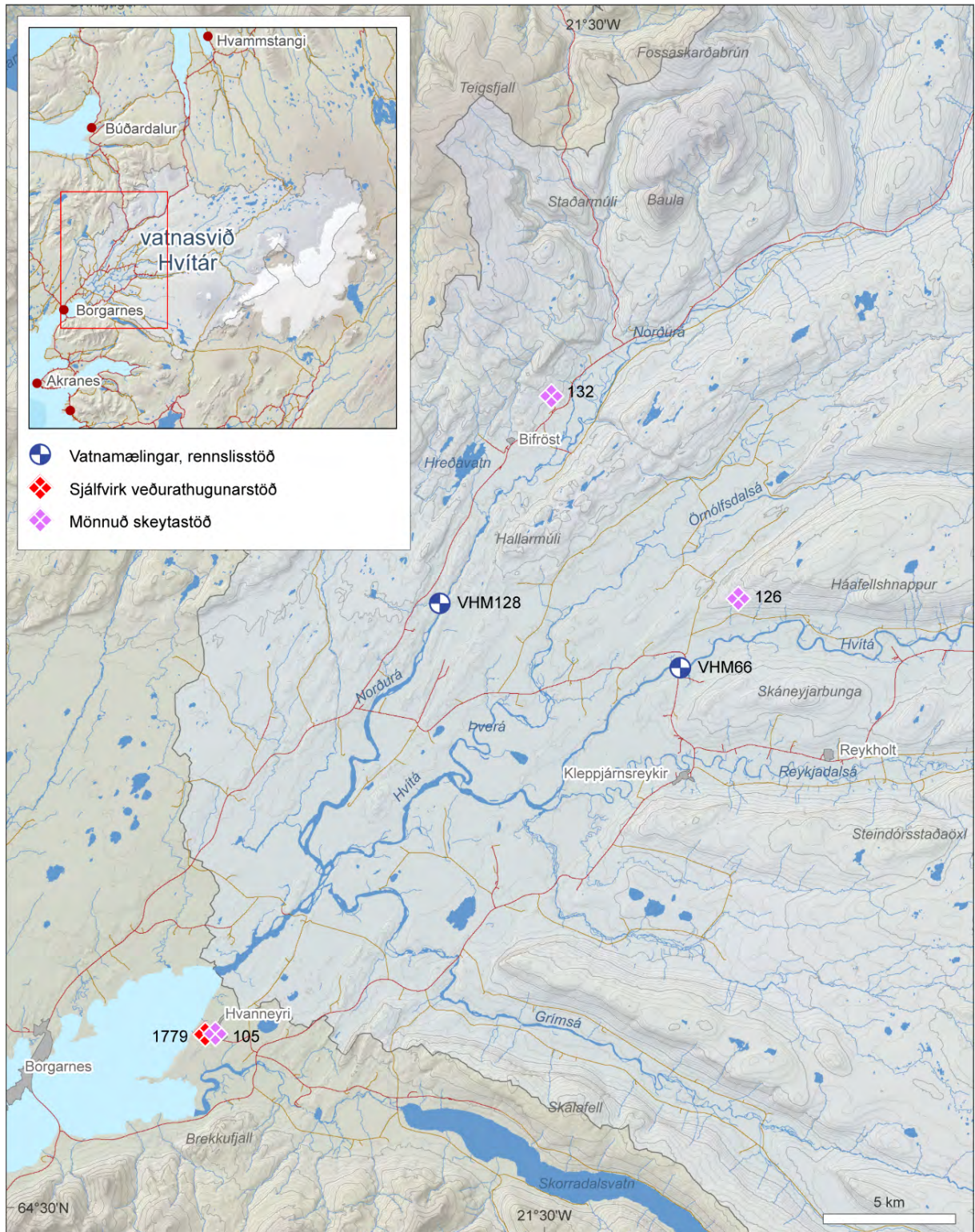
Mynd IV-2. Staðsetning veðurstöðva og vatnshæðarmæla sem notaðar voru til að greina og flokka flóðaatburði á vatnasviði Hvítár.
