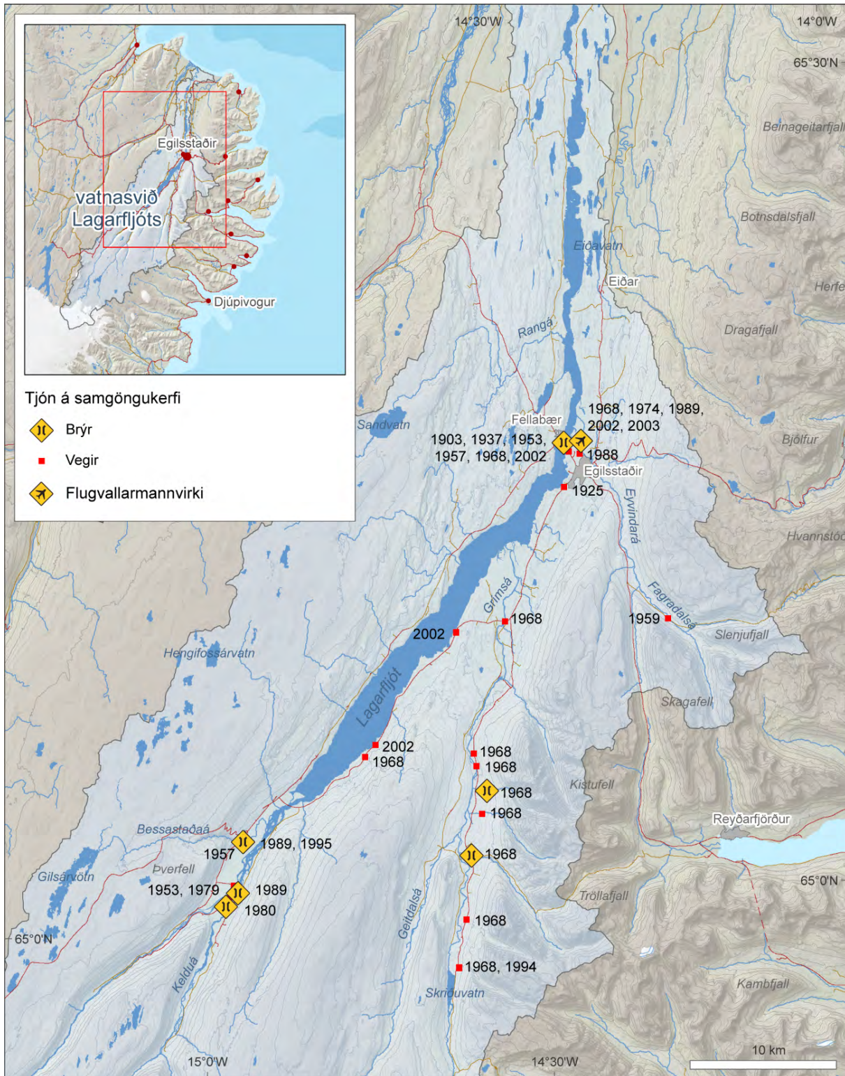
Mynd V-9. Tjón á samgöngukerfinu af völdum flóða á vatnasviði Lagarfljóts.
