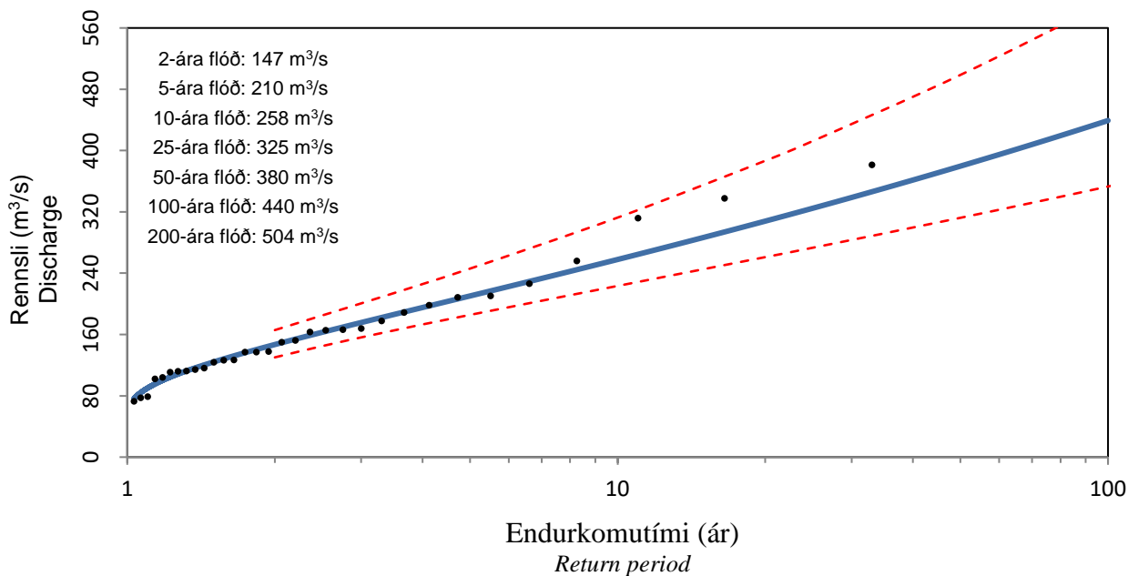
Reiknuð og mæld hæstu flóð árána 1985–2016 ásamt 95% öryggisbili Calculated and measured maximum floods with 95% confidence interval
