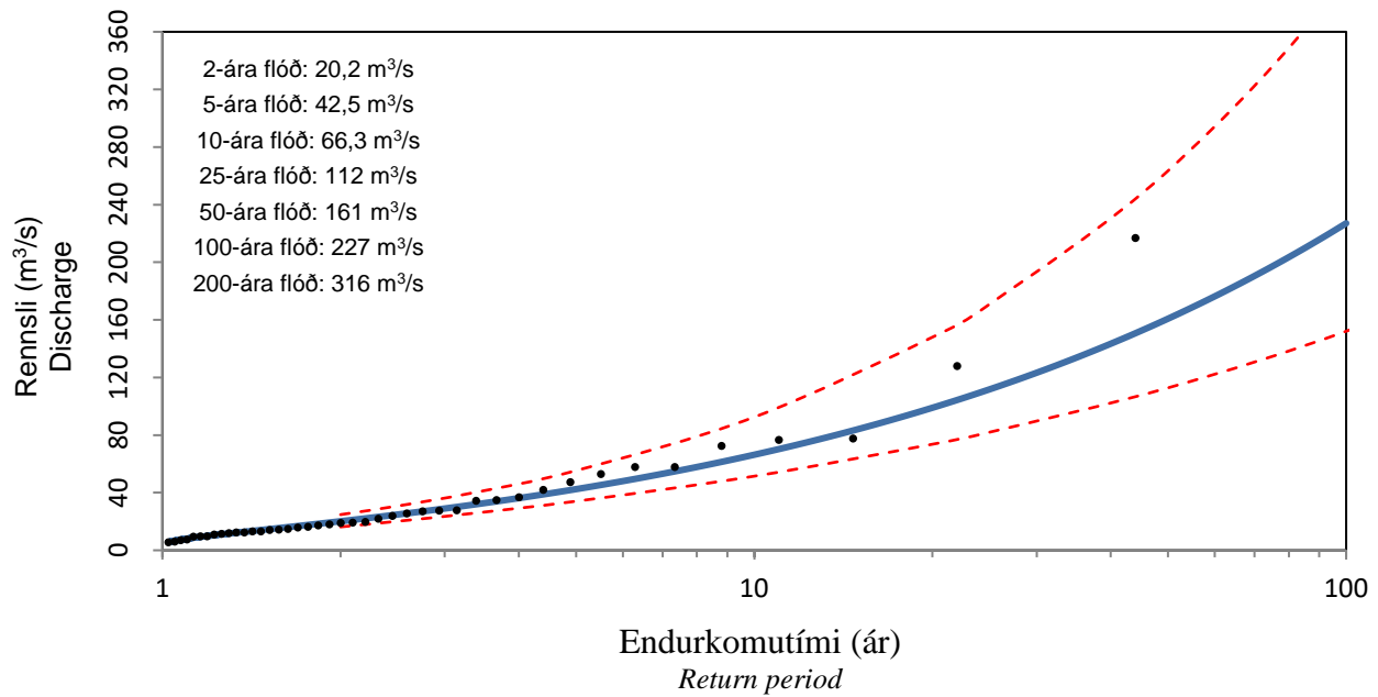
Reiknuð og mæld hæstu flóð árána 1974-2016 ásamt 95% öryggisbili Calculated and measured maximum floods with 95% confidence interval
