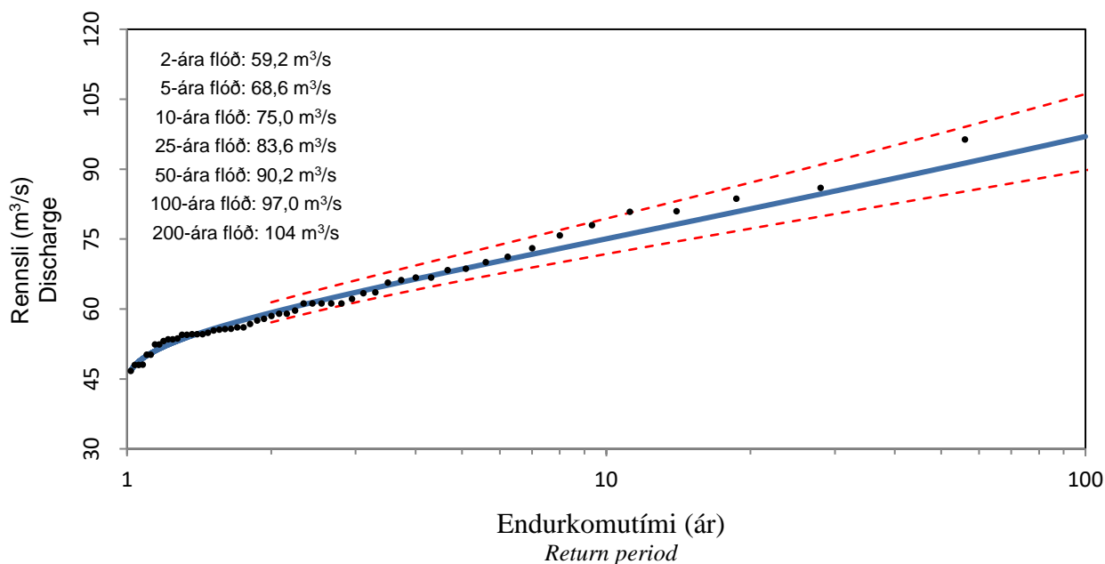
Reiknuð og mæld hæstu flóð árána 1962-2016 ásamt 95% öryggisbili Calculated and measured maximum floods with 95% confidence interval
