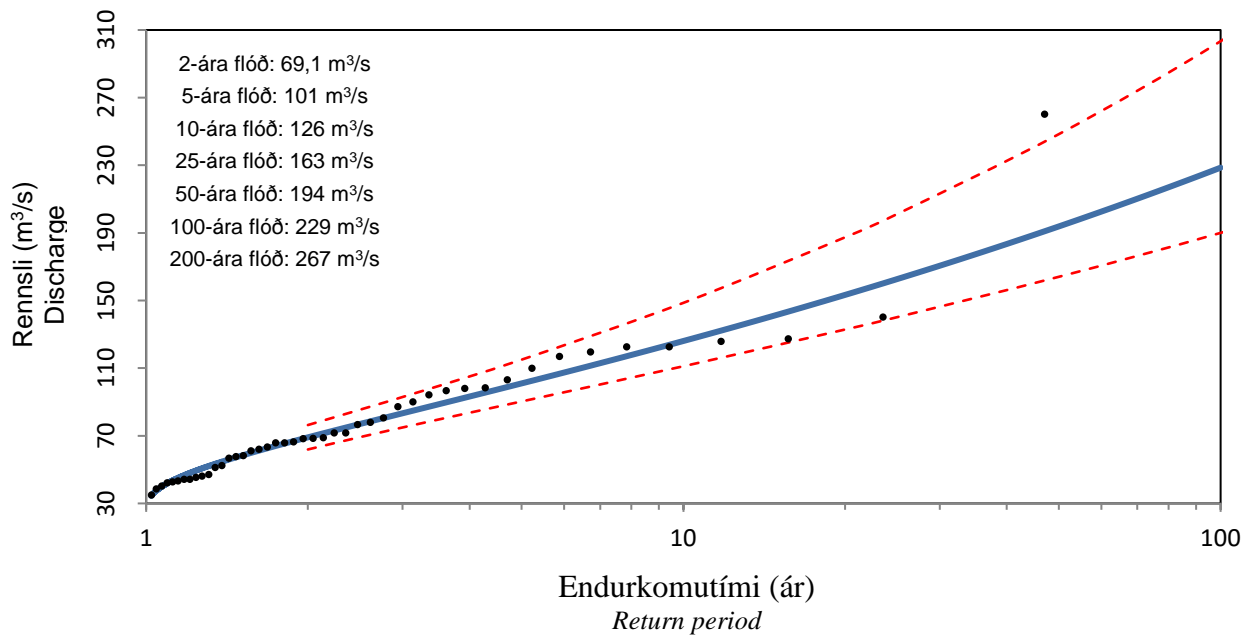
Reiknuð og mæld hæstu flóð árána 1971-2016 ásamt 95% öryggisbili Calculated and measured maximum floods with 95% confidence interval
