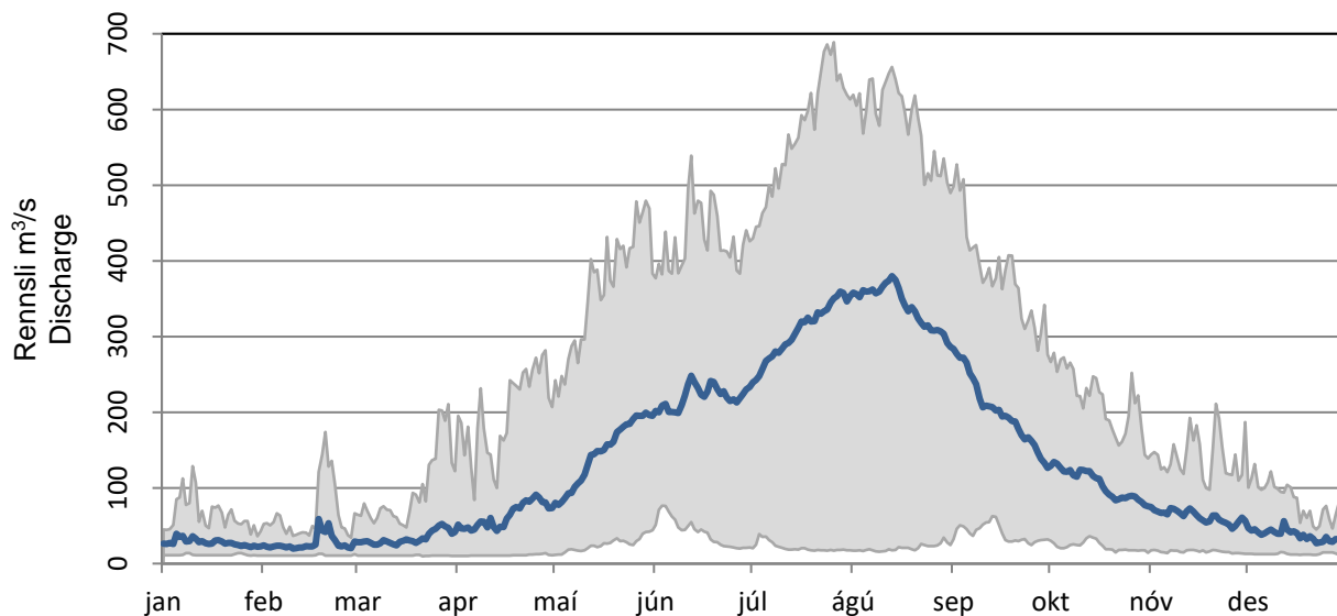
Miðgildi dagsmeðalrennslis ásamt 95% og 5% hlutfallsmörkum Long term median of daily averages and 95 th and 5 th percentiles
