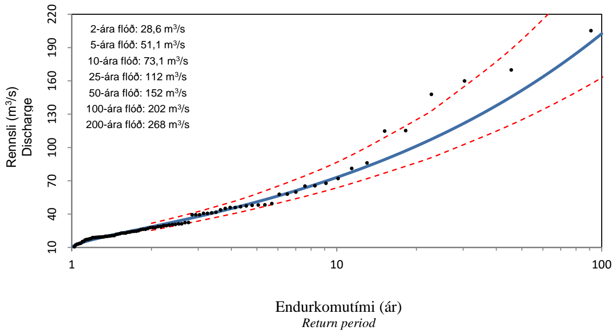
Reiknuð og mæld hæstu flóð árána 1927-2016 ásamt 95% öryggisbili Calculated and measured maximum floods with 95% confidence interval
