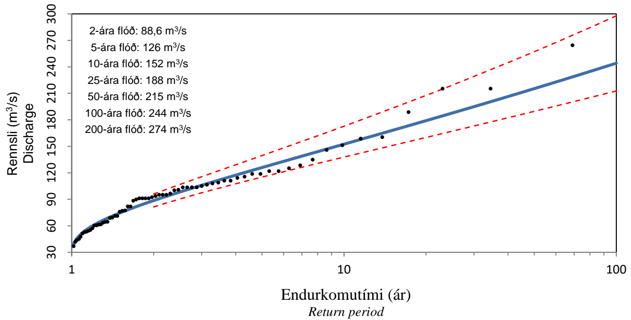
Reiknuð og mæld hæstu flóð árána 1949-2016 ásamt 95% öryggisbili Calculated and measured maximum floods with 95% confidence interval
