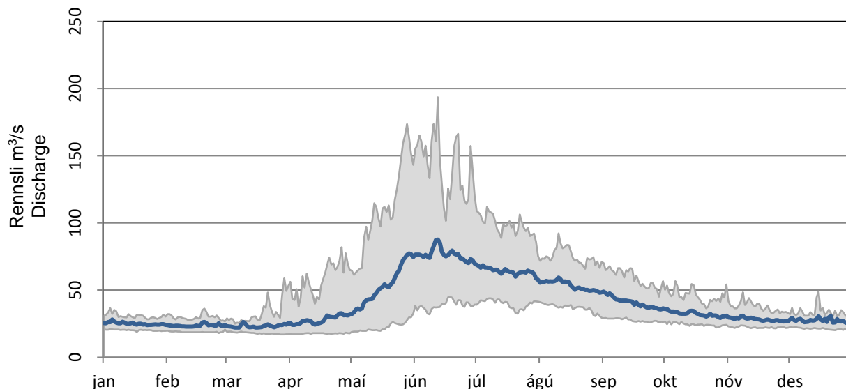
Miðgildi dagsmeðalrennslis ásamt 95% og 5% hlutfallsmörkum Median daily averages and 95 th and 5 th percentiles
