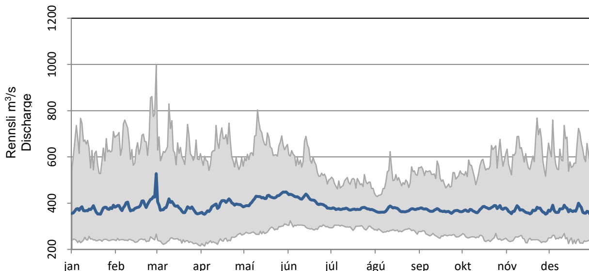
Miðgildi dagsmeðalrennsli ásamt 95% og 5% hlutfallsmörkum Median of daily averages and 95 th and 5 th percentiles
