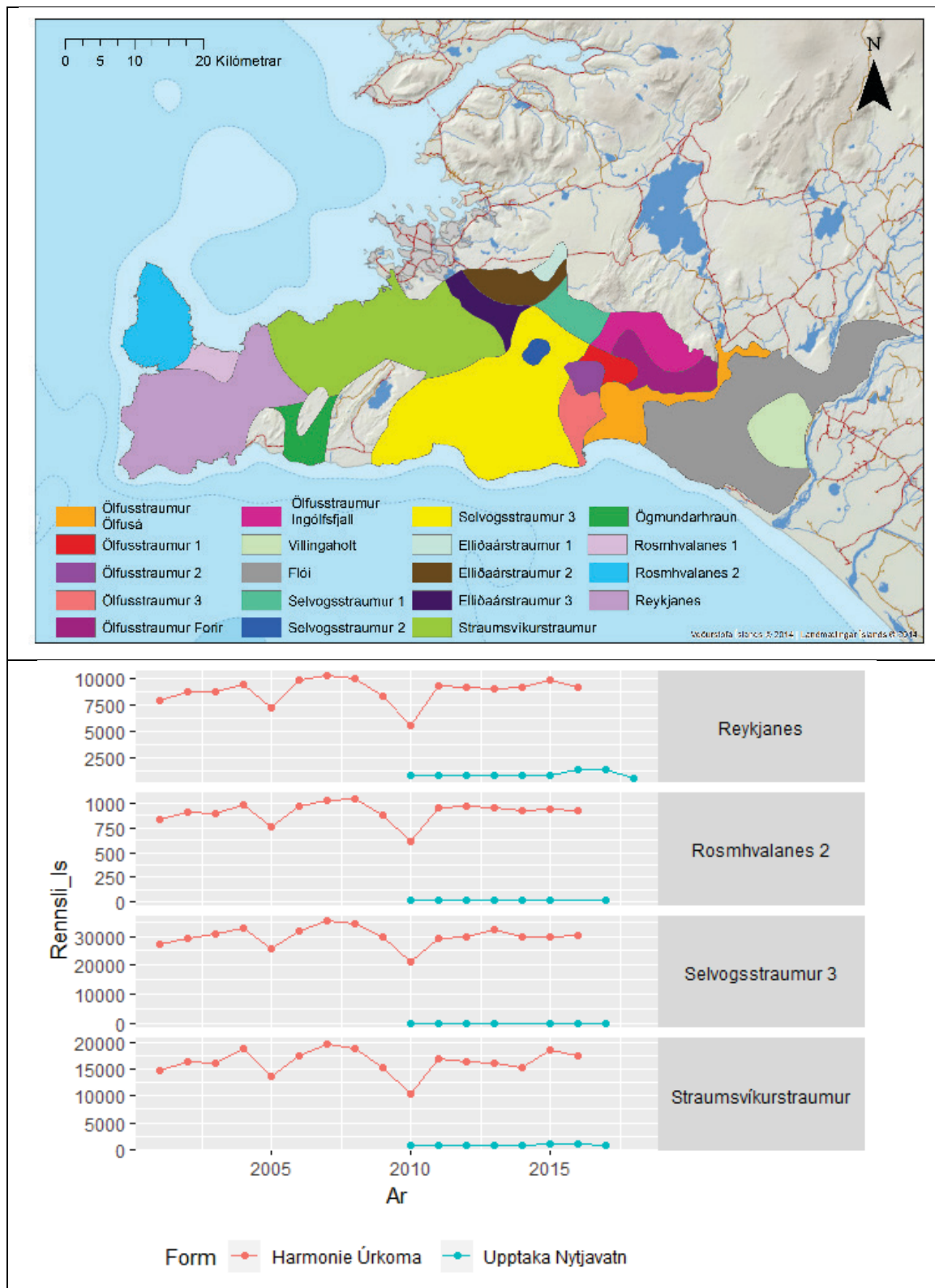
Mynd 6. Vatnstaka úr grunnvatnshlotum á Reykjanesi samkvæmt upplýsingum úr Nytjavatnsgrunni. Samanburður á úrkomu og upptöku vatns í þeim hlotum sem mest er tekið úr. Vatnstaka úr Selvogsstraumi 3 er að öllum líkindum verulega vanáætluð.
