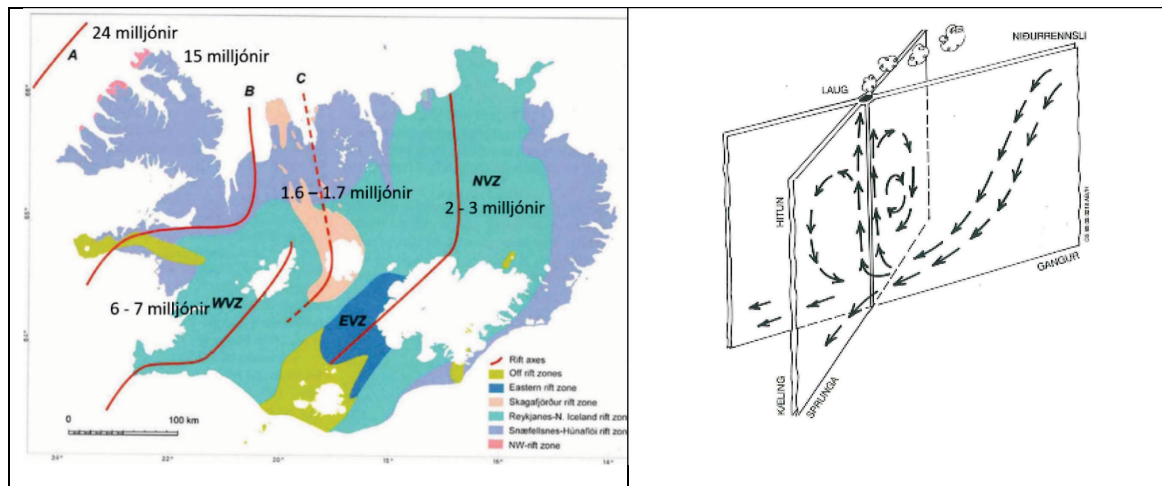
Mynd 37. Jarðhiti og landrek: a) Færsla rekbeltanna á Íslandi í gegnum tíðina (Björn S. Harðarson o.fl., 2008); b) Lágðitasvæðin eru gjarnan tengd tveimur sprungukerfum með mismunandi stefnu. Þar sem sprungurnar skerast er lektin mest og heita vatnið leitar þar til yfirborðs (Axel Björnsson, 1989).
