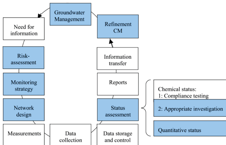
Mynd 4. Rannsóknarferli við stýringu grunnvatnsnýtingar. Bláu kassarnir sýna hvar hugtakalíkonin (CM = Conceptual Model) eru gagnleg eða jafnvel nauðsynleg (European Commission Environment, 2010).
