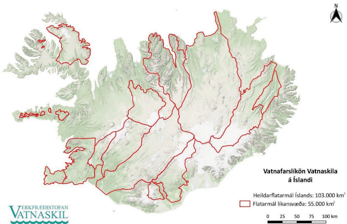
Mynd 9. Þau landsvæði sem vatnafarslíkön með grunnvatni ná yfir (Vatnaskil, 2019).
