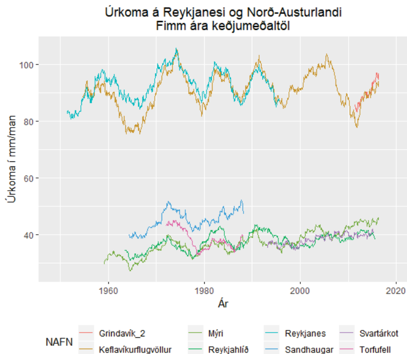
Mynd 12. Mánaðarúrkoma á SV og NA landi síðustu 50 ár. Fimm ára keðjumeðaltöl (Veðurstofa Íslands, 2019).
