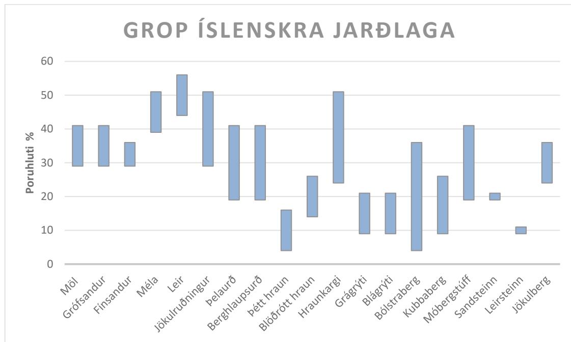
Mynd 20. Grop íslenskra jarðefna (Árni Hjartarson, 1993).
