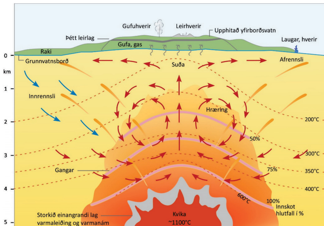
Mynd 35. Einfaldað þversnið af háhitavæði. Háhitavæði myndast við staðbundna hringrás vatns í sprungnu bergi yfir kvikuhólfu eða kólnandi innskoti sem er á fátíðum kílómetra dýpi í jarðskorpunni (Stefán Arnórsson, 2011).
