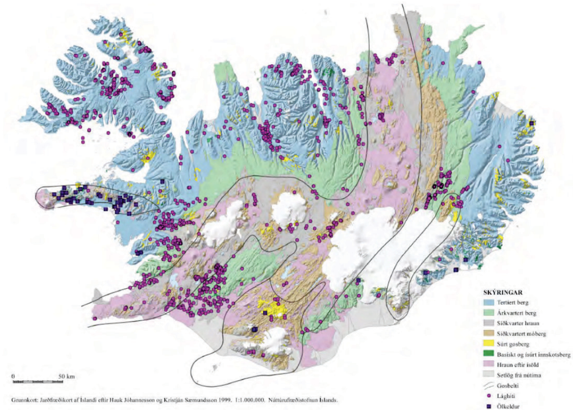
Mynd 36. Lághiti og ölkeldur á Íslandi (Stefán Arnórsson, 2011).
