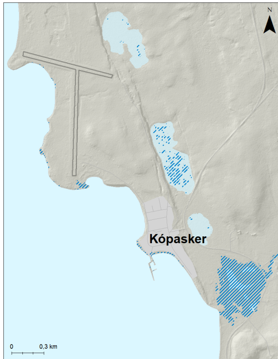
Mynd 214. Kópasker. Möguleg útbreiðsla sjávarflóðs sem hefur 20 ára endurkomutíma (5% árslíkur) árið 2100 miðað við sviðsmynd SSP5-8.5.
