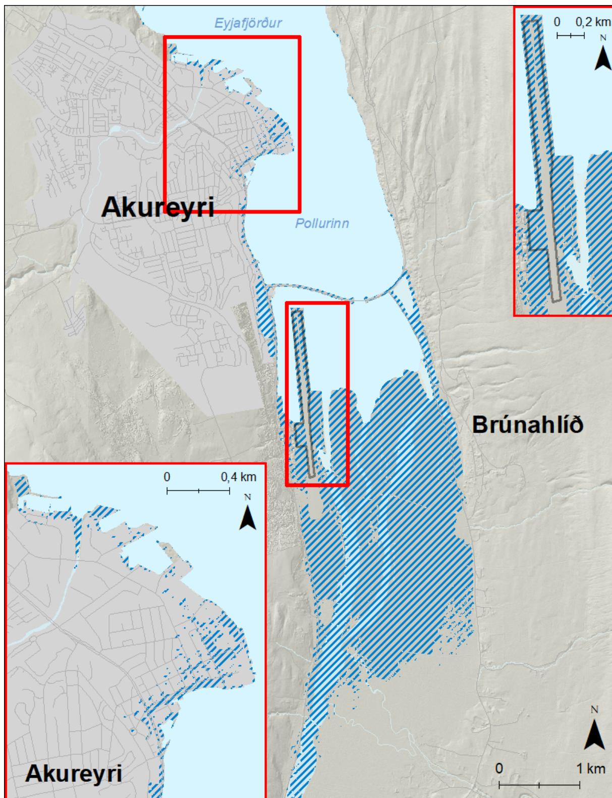
Mynd 131. Akureyri. Möguleg útbreiðsla sjávarflóðs sem hefur 200 ára endurkomutíma (0,5% árslíkur) við núverandi aðstæður.
