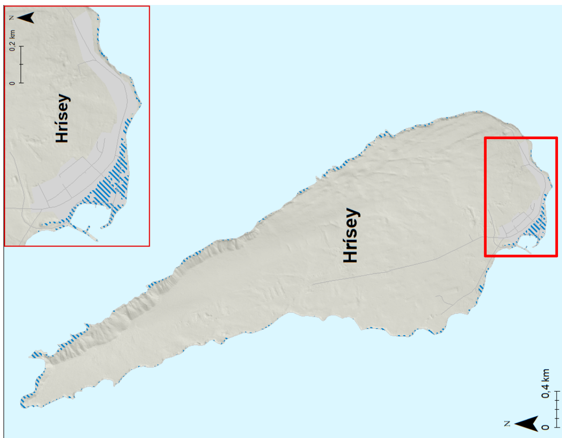
Mynd 56. Hrísey. Möguleg úbreiðsla sjávarflóðs sem hefur 50 ára endurkomutíma (0,5% árslíkur) árið 2150 miðað við sviðsmynd SSP5-8.5LC.
