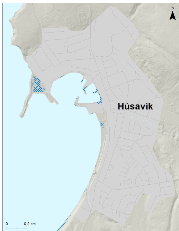
Mynd 200. Húsavík. Möguleg útbreiðsla sjávarflóðs sem hefur 20 ára endurkomutíma (5% árslíkur) árið 2150 miðað við sviðsmynd SSP5-8.5.
