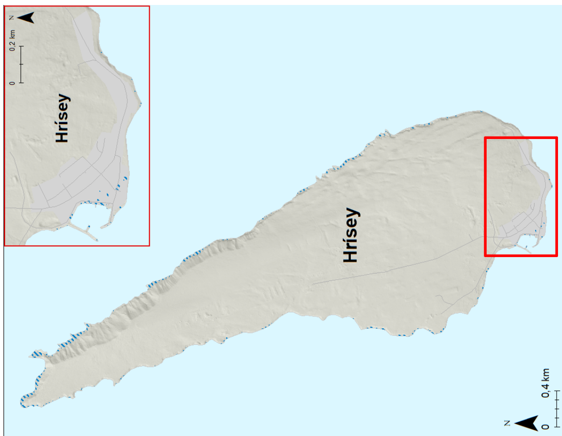
Mynd 46. Hrísey. Möguleg útbreiðsla sjávarflóðs sem hefur 20 ára endurkomutíma (5% árslíkur) við núverandi aðstæður.
