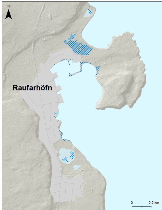
Mynd 226. Raufarhöfn. Möguleg útbreiðsla sjávarflóðs sem hefur 20 ára endurkomutíma (5% árslíkur) við núverandi aðstæður.
