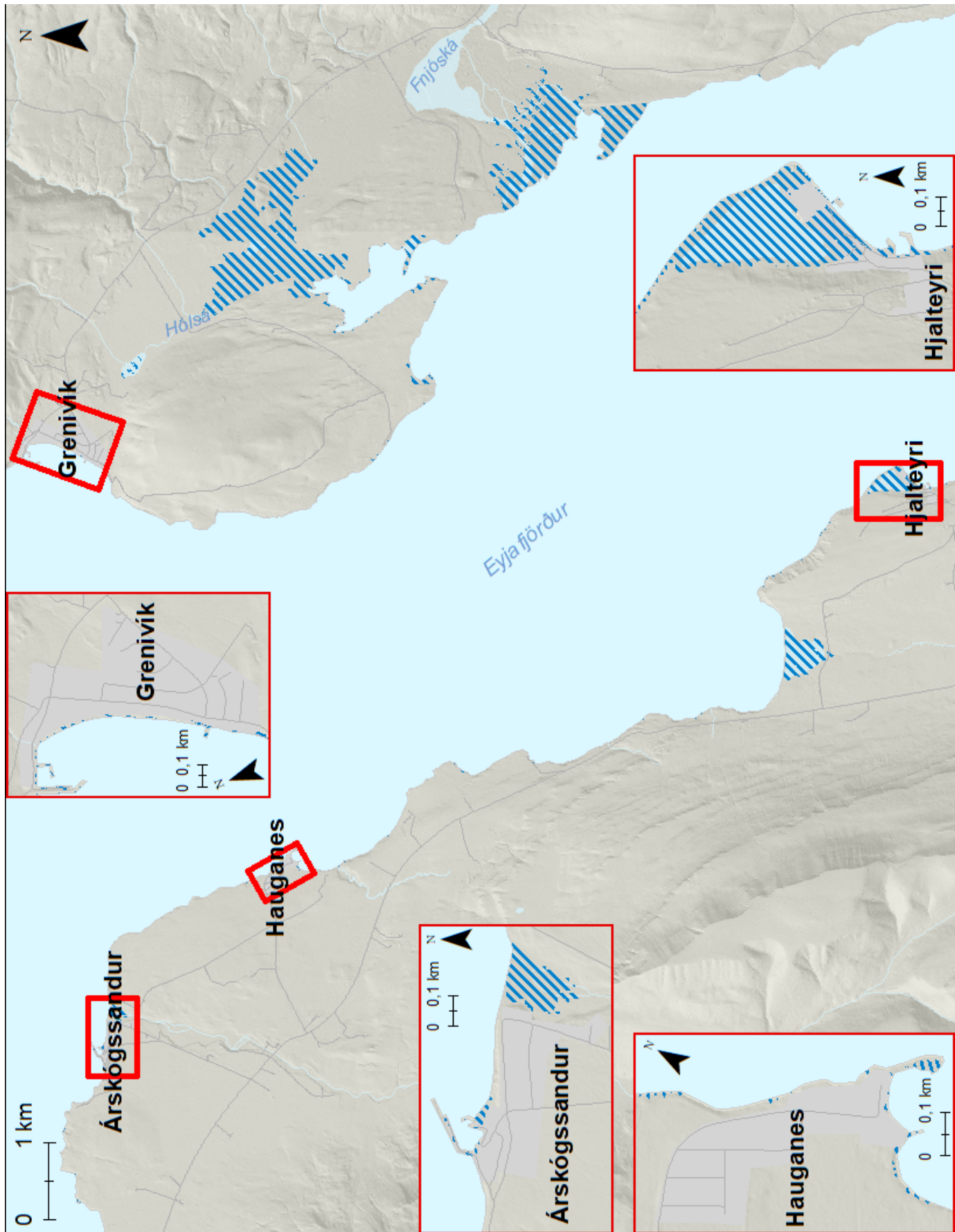
Mynd 68. Árskógssandur, Grenivík, Hauganes og Hjalteyri. Möguleg útbreiðsla sjávarflóðs sem hefur 50 ára endurkomutíma (2% árslíkur) árið 2100 miðað við sviðsmynd SSP5-8.5LC.
