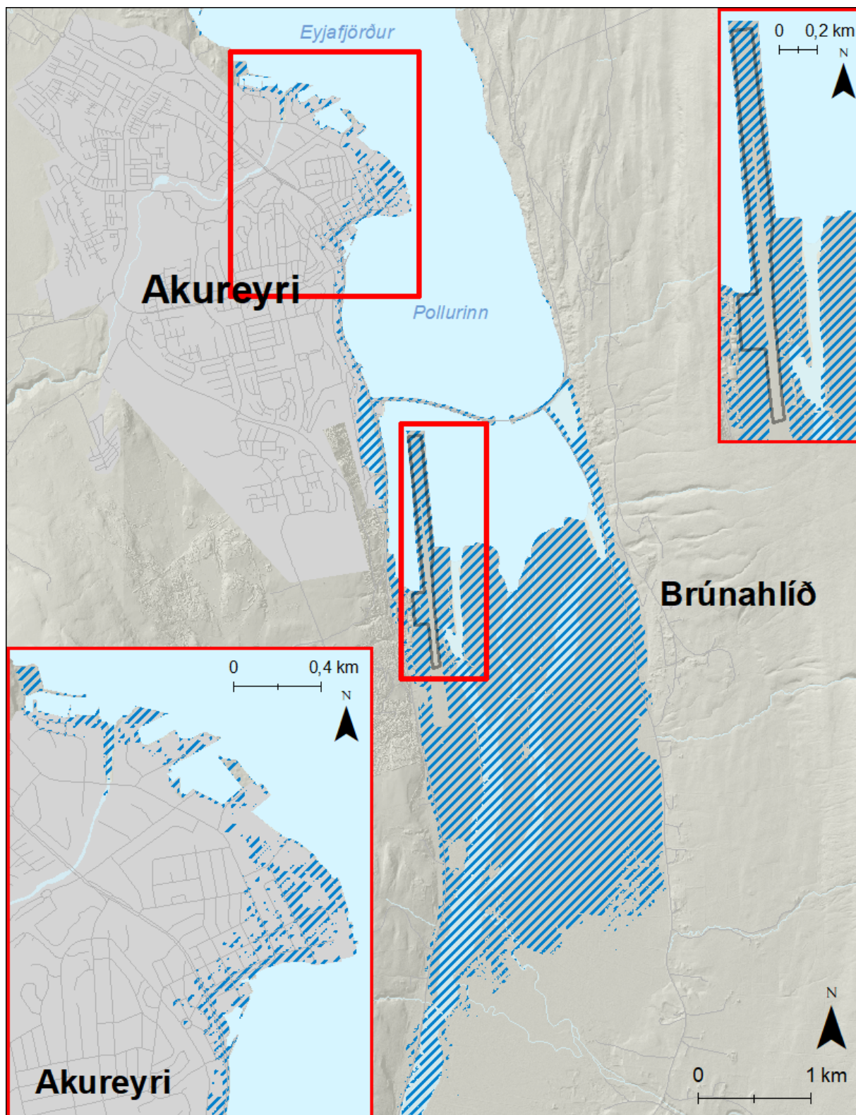
Mynd 128. Akureyri. Möguleg útbreiðsla sjávarflóðs sem hefur 50 ára endurkomutíma (2% árslíkur) árið 2100 miðað við sviðsmynd SSP5-8.5LC.
