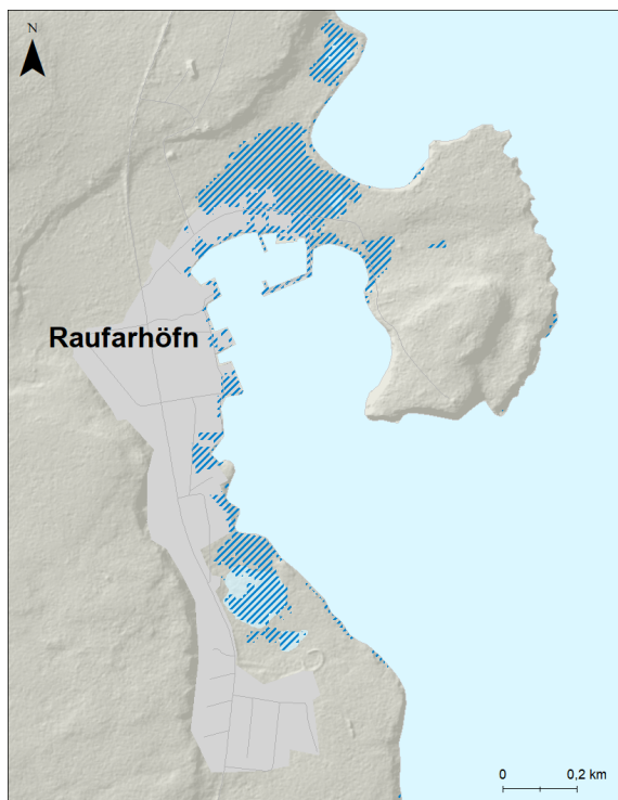
Mynd 234. Raufarhöfn. Möguleg útbreiðsla sjávarflóðs sem hefur 50 ára endurkomutíma (2% árslíkur) árið 2150 miðað við sviðsmynd SSP5-8.5.
