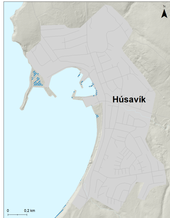
Mynd 198. Húsavík. Möguleg útbreiðsla sjávarflóðs sem hefur 200 ára endurkomutíma (0,5% árslíkur) við núverandi aðstæður.
