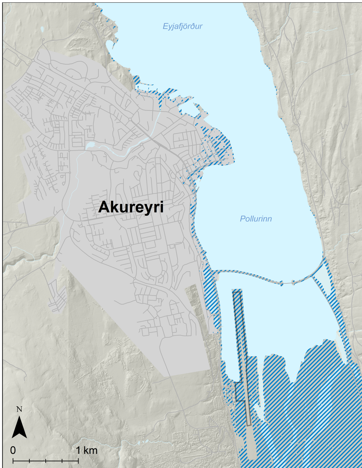
Mynd 149. Akureyri. Möguleg útbreiðsla sjávarflóðs sem hefur 200 ára endurkomutíma (0,5% árslíkur) árið 2150 miðað við sviðsmynd SSP5-8.5.
