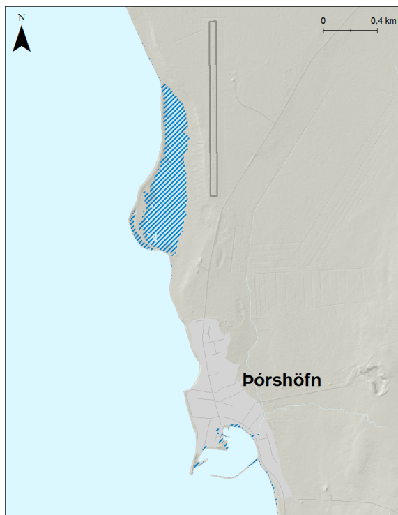
Mynd 249. Þórshöfn. Möguleg útbreiðsla sjávarflóðs sem hefur 50 ára endurkomutíma (2% árslíkur) árið 2150 miðað við sviðsmynd SSP5-8.5.
