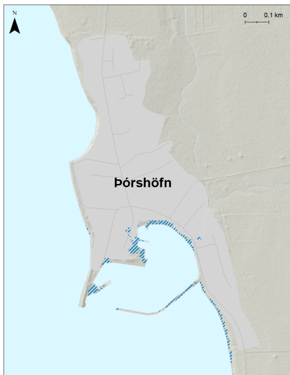
Mynd 264. Þórshöfn. Möguleg útbreiðsla sjávarflóðs sem hefur 50 ára endurkomutíma (2% árslíkur) árið 2150 miðað við sviðsmynd SSP5-8.5.
