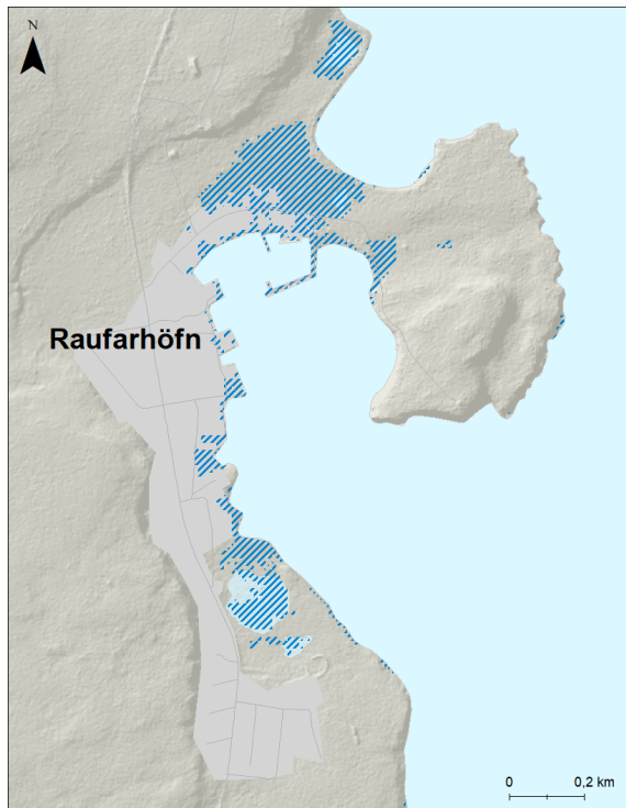
Mynd 230. Raufarhöfn. Möguleg útbreiðsla sjávarflóðs sem hefur 20 ára endurkomutíma (5% árslíkur) árið 2150 miðað við sviðsmynd SSP5-8.5.
