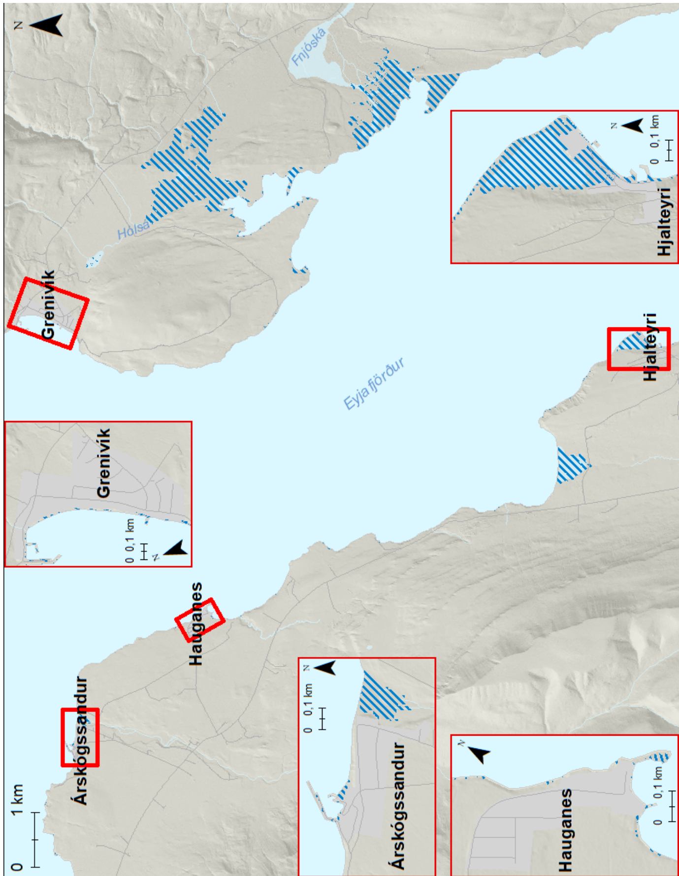
Mynd 63. Árskógssandur, Grenivík, Hauganes og Hjalteyri. Möguleg útbreiðsla sjávarflóðs sem hefur 20 ára endurkomutíma (5% árslíkur) árið 2100 miðað við sviðsmynd SSP5-8.5LC.
