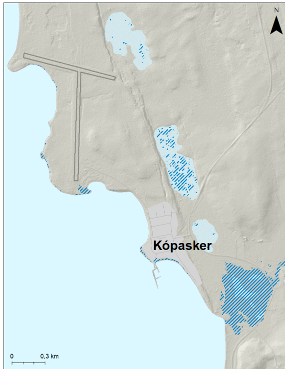
Mynd 218. Kópasker. Möguleg útbreiðsla sjávarflóðs sem hefur 50 ára endurkomutíma (2% árslíkur) árið 2100 miðað við sviðsmynd SSP5-8.5.
