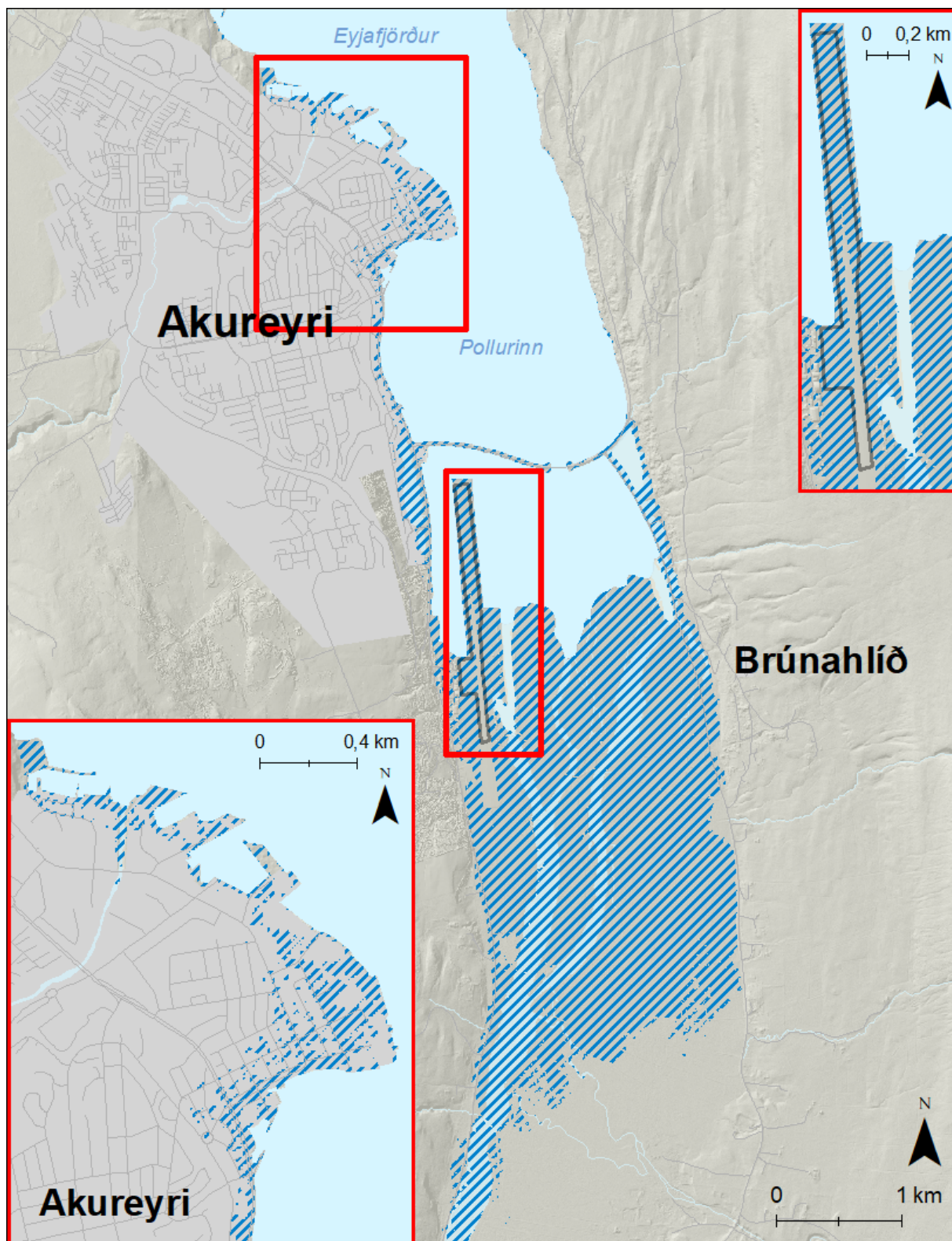
Mynd 133. Akureyri. Möguleg útbreiðsla sjávarflóðs sem hefur 200 ára endurkomutíma (0,5% árslíkur) árið 2100 miðað við sviðsmynd SSP5-8.5LC.
