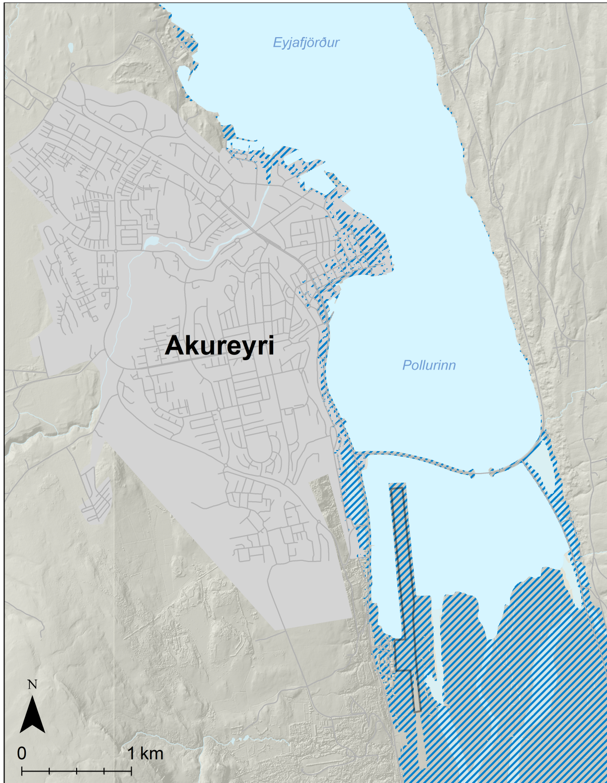
Mynd 145. Akureyri. Möguleg útbreiðsla sjávarflóðs sem hefur 50 ára endurkomutíma (2% árslíkur) árið 2150 miðað við sviðsmynd SSP5-8.5LC.
