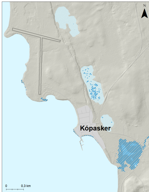
Mynd 212. Kópasker. Möguleg útbreiðsla sjávarflóðs sem hefur 50 ára endurkomutíma (2% árslíkur) við núverandi aðstæður.
