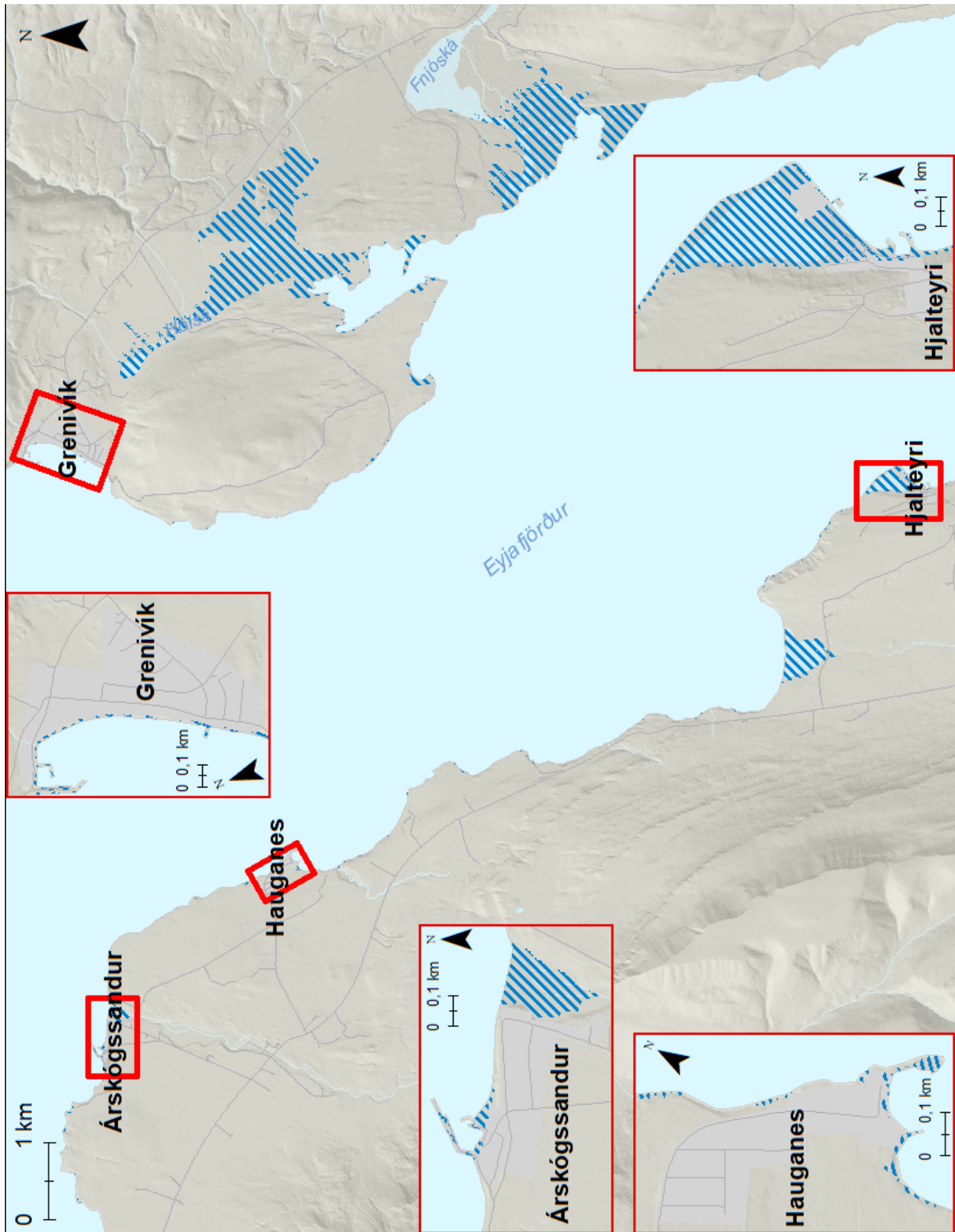
Mynd 70. Árskógssandur, Grenivík, Hauganes og Hjalteyri. Möguleg útbreiðsla sjávarflóðs sem hefur 50 ára endurkomutíma (2% árslíkur) árið 2150 miðað við sviðsmynd SSP5-8.5LC.
