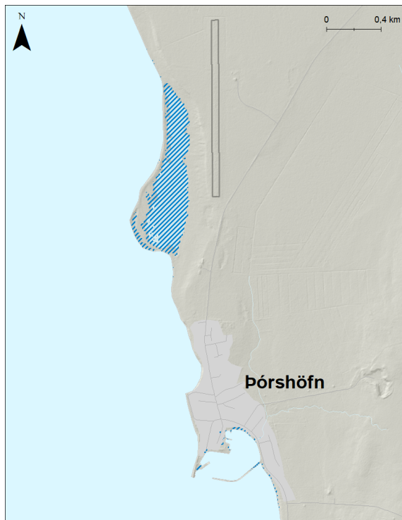
Mynd 248. Þórshöfn. Möguleg útbreiðsla sjávarflóðs sem hefur 50 ára endurkomutíma (2% árslíkur) árið 2100 miðað við sviðsmynd SSP5-8.5.
