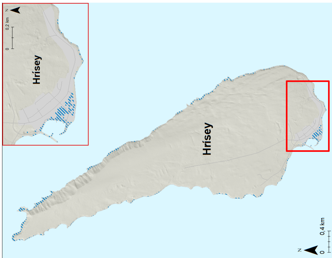
Mynd 55. Hrísey. Möguleg úbreiðsla sjávarflóðs sem hefur 50 ára endurkomutíma (0,5% árslíkur) árið 2100 miðað við sviðsmynd SSP5-8.5LC.
