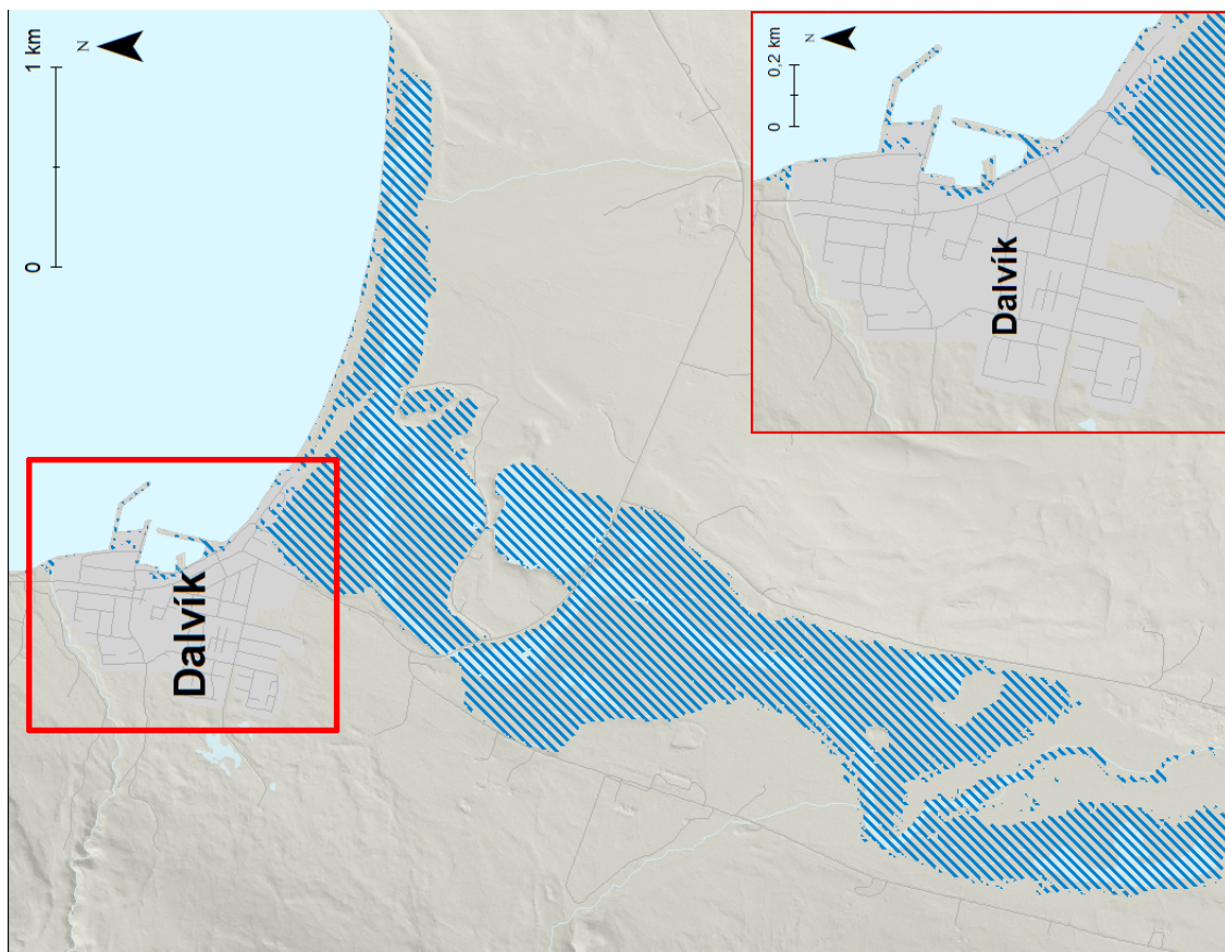
Mynd 39. Dalvík. Möguleg útbreiðsla sjávarflóðs sem hefur 200 ára endurkomutíma (0,5% árslíkur) árið 2100 miðað við sviðsmynd SSP5-8.5.
