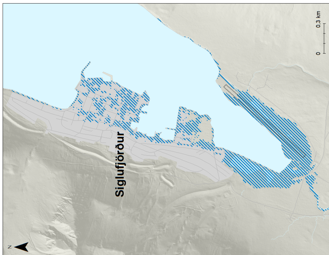
Mynd 5. Siglufjörður. Möguleg útbreiðsla sjávarflóðs sem hefur 50 ára endurkomutíma (0,5% árslíkur) árið 2100 miðað við sviðsmynd SSP5-8.5.
