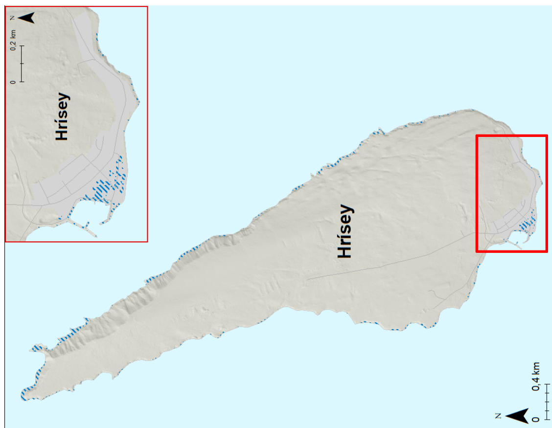
Mynd 49. Hrísey. Möguleg úbreiðsla sjávarflóðs sem hefur 20 ára endurkomutíma (0,5% árslíkur) árið 2100 miðað við sviðsmynd SSP5-8.5.
