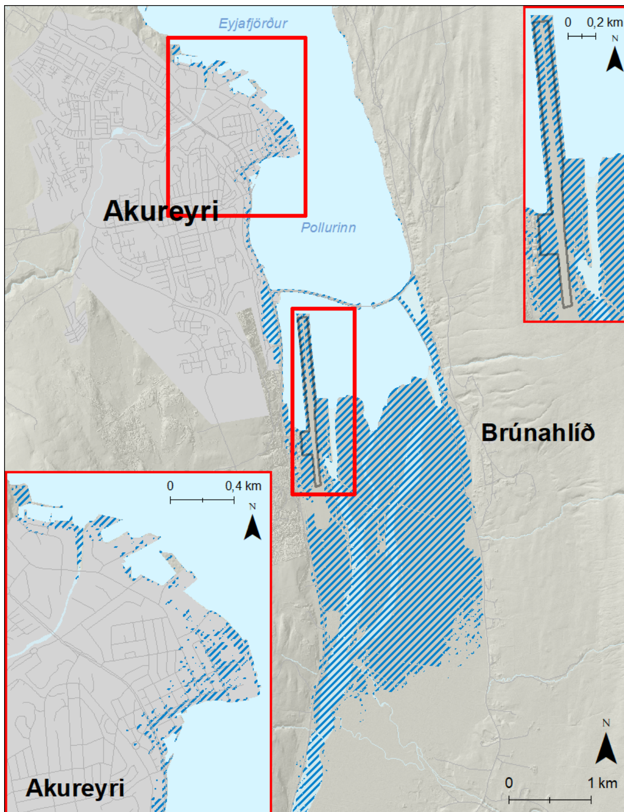
Mynd 127. Akureyri. Möguleg útbreiðsla sjávarflóðs sem hefur 50 ára endurkomutíma (2% árslíkur) árið 2100 miðað við sviðsmynd SSP5-8.5.
