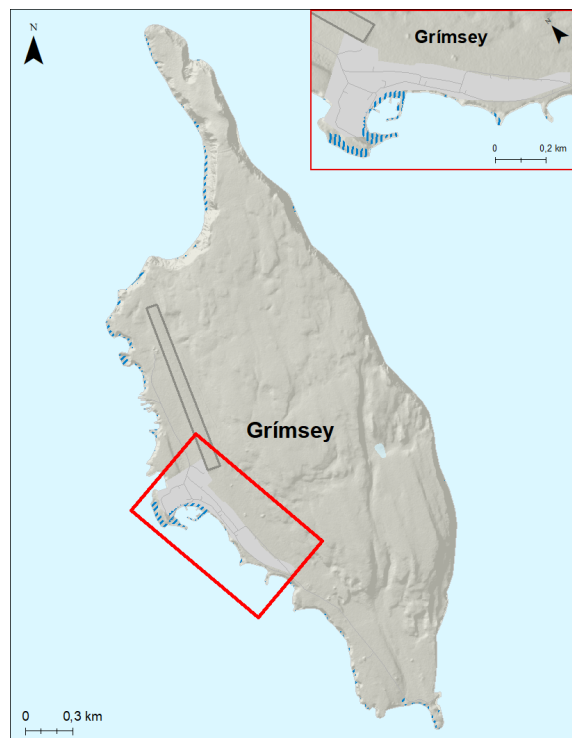
Mynd 187. Grímsey. Möguleg útbreiðsla sjávarflóðs sem hefur 20 ára endurkomutíma (5% árslíkur) árið 2150 miðað við sviðsmynd SSP5-8.5LC.
