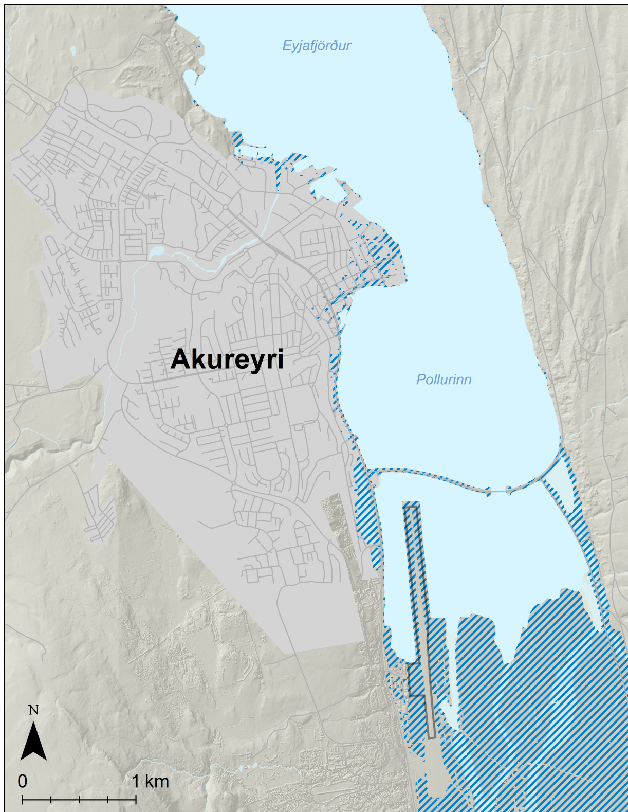
Mynd 139. Akureyri. Möguleg útbreiðsla sjávarflóðs sem hefur 20 ára endurkomutíma (5% árslíkur) árið 2150 miðað við sviðsmynd SSP5-8.5.
