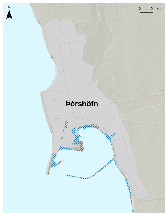
Mynd 262. Þórshöfn. Möguleg útbreiðsla sjávarflóðs sem hefur 20 ára endurkomutíma (5% árslíkur) árið 2150 miðað við sviðsmynd SSP5-8.5LC.
