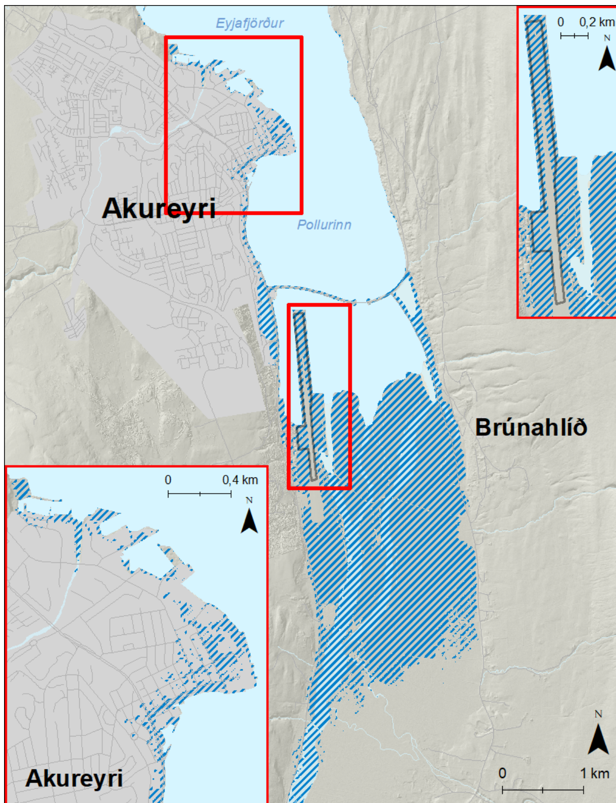
Mynd 123. Akureyri. Möguleg útbreiðsla sjávarflóðs sem hefur 20 ára endurkomutíma (5% árslíkur) árið 2100 miðað við sviðsmynd SSP5-8.5LC.
