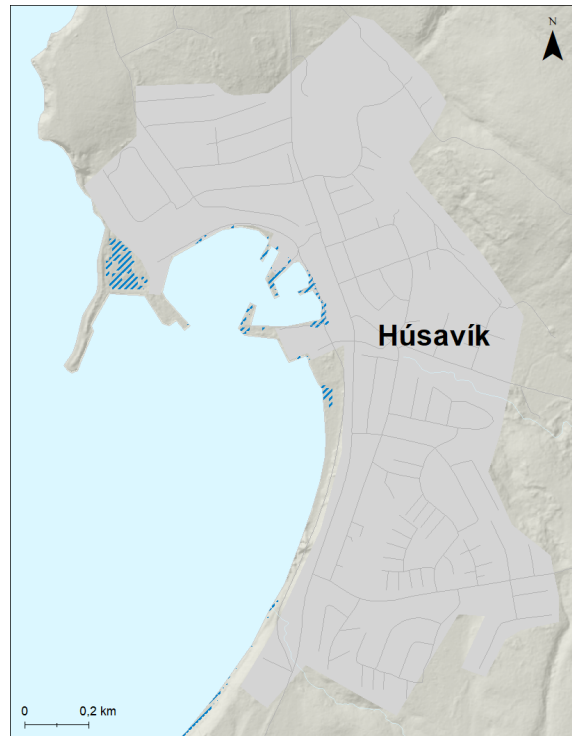
Mynd 205. Húsavík. Möguleg útbreiðsla sjávarflóðs sem hefur 50 ára endurkomutíma (2% árslíkur) árið 2100 miðað við sviðsmynd SSP5-8.5LC.
