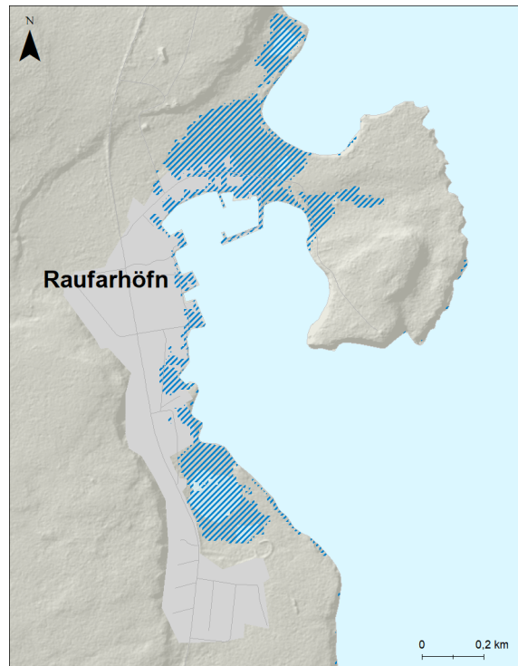
Mynd 232. Raufarhöfn. Möguleg útbreiðsla sjávarflóðs sem hefur 20 ára endurkomutíma (5% árslíkur) árið 2150 miðað við sviðsmynd SSP5-8.5LC.
