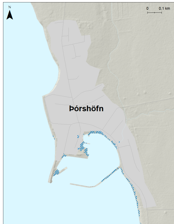
Mynd 261. Þórshöfn. Möguleg útbreiðsla sjávarflóðs sem hefur 20 ára endurkomutíma (5% árslíkur) árið 2100 miðað við sviðsmynd SSP5-8.5LC.
