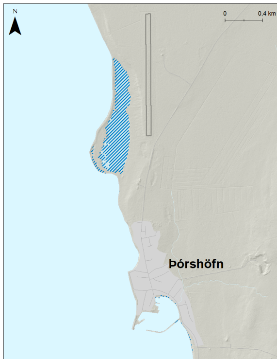
Mynd 241. Þórshöfn. Möguleg útbreiðsla sjávarflóðs sem hefur 20 ára endurkomutíma (5% árslíkur) við núverandi aðstæður.
