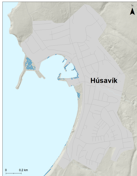
Mynd 209. Húsavík. Möguleg útbreiðsla sjávarflóðs sem hefur 200 ára endurkomutíma (0,5% árslíkur) árið 2100 miðað við sviðsmynd SSP5-8.5LC.
