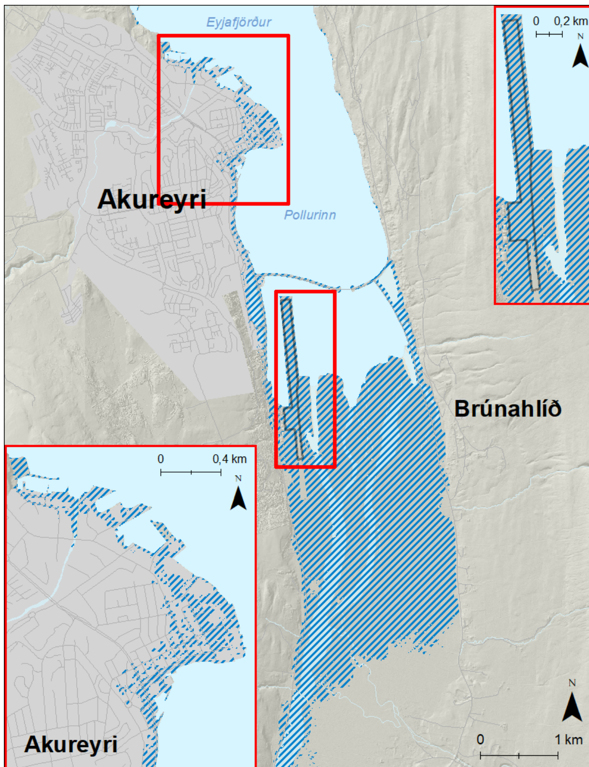
Mynd 130. Akureyri. Möguleg útbreiðsla sjávarflóðs sem hefur 50 ára endurkomutíma (2% árslíkur) árið 2150 miðað við sviðsmynd SSP5-8.5LC.
