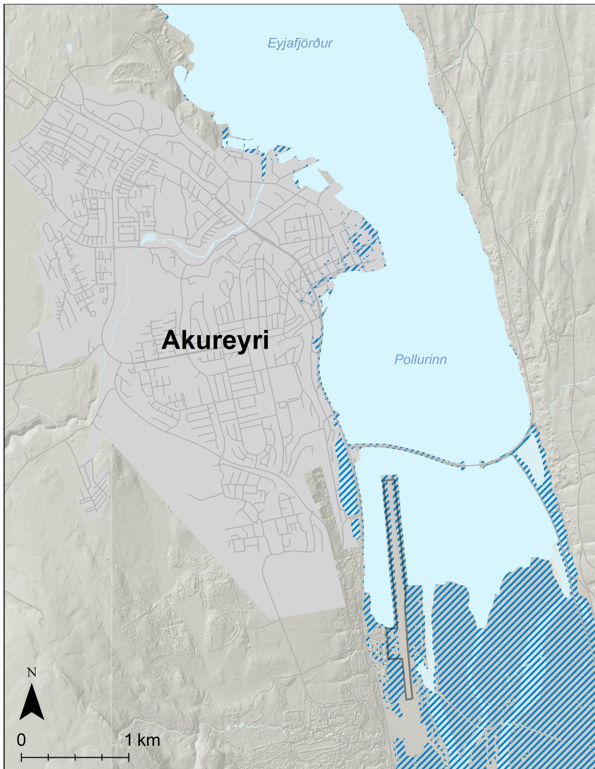
Mynd 136. Akureyri. Möguleg útbreiðsla sjávarflóðs sem hefur 20 ára endurkomutíma (5% árslíkur) við núverandi aðstæður.
