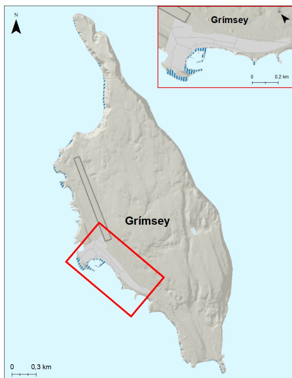
Mynd 189. Grímsey. Möguleg útbreiðsla sjávarflóðs sem hefur 50 ára endurkomutíma (2% árslíkur) árið 2150 miðað við sviðsmynd SSP5-8.5.
