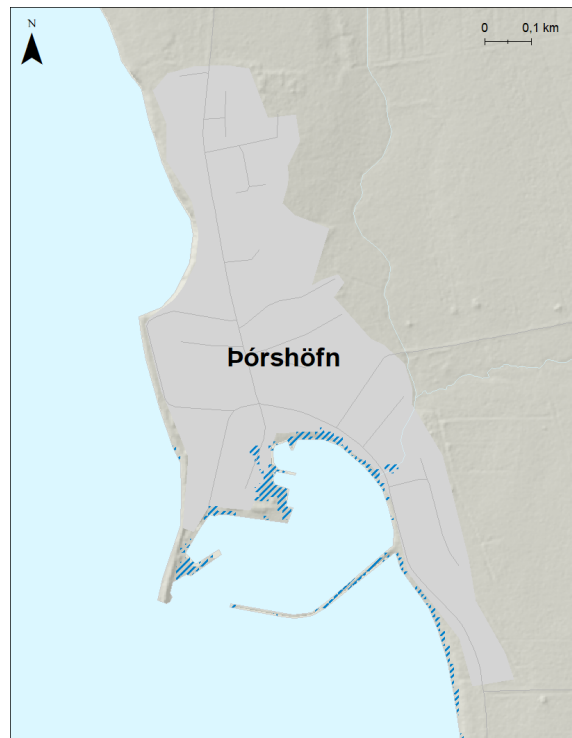
Mynd 269. Þórshöfn. Möguleg útbreiðsla sjávarflóðs sem hefur 200 ára endurkomutíma (0,5% árslíkur) árið 2100 miðað við sviðsmynd SSP5-8.5LC.
