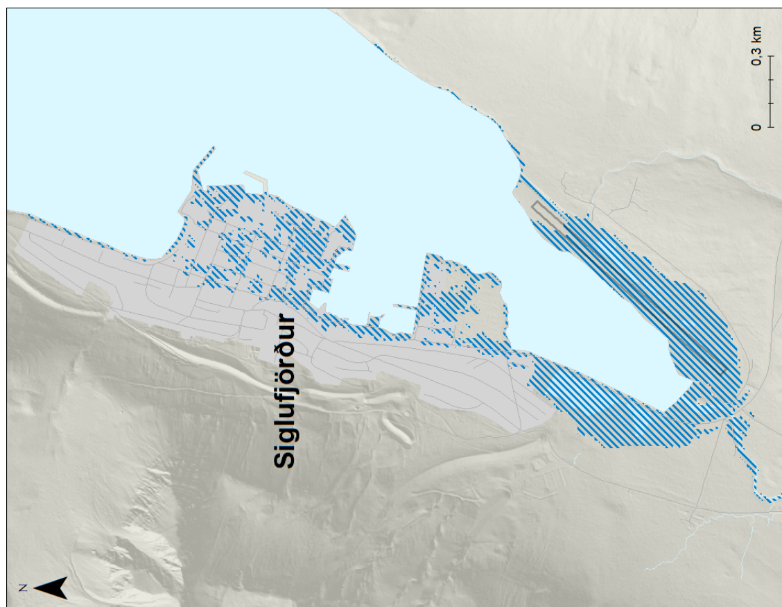
Mynd 1. Siglufjörður. Möguleg útbreiðsla sjávarflóðs sem hefur 20 ára endurkomutíma (0,5% árslíkur) árið 2100 miðað við sviðsmynd SSP5-8.5.
