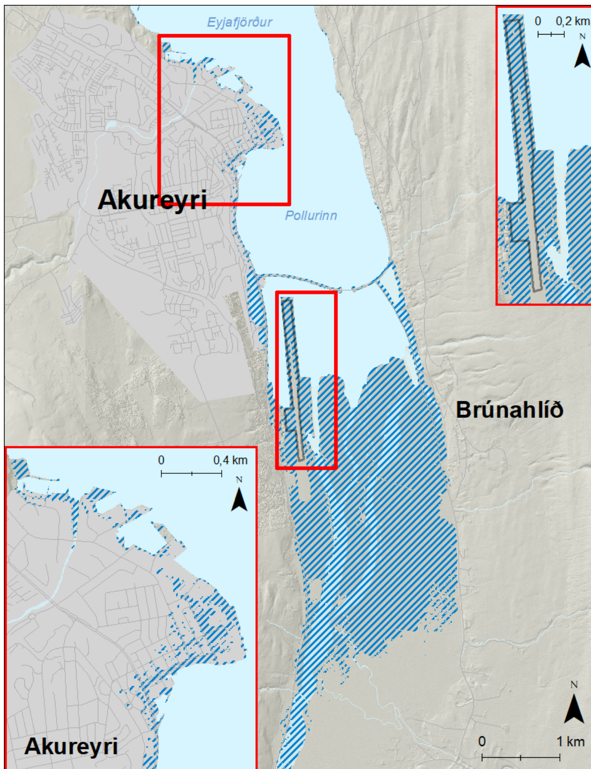
Mynd 132. Akureyri. Möguleg útbreiðsla sjávarflóðs sem hefur 200 ára endurkomutíma (0,5% árslíkur) árið 2100 miðað við sviðsmynd SSP5-8.5.
