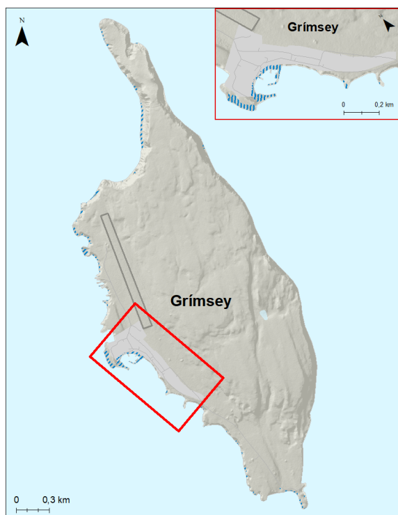
Mynd 193. Grímsey. Möguleg útbreiðsla sjávarflóðs sem hefur 200 ára endurkomutíma (0,5% árslíkur) árið 2150 miðað við sviðsmynd SSP5-8.5.
