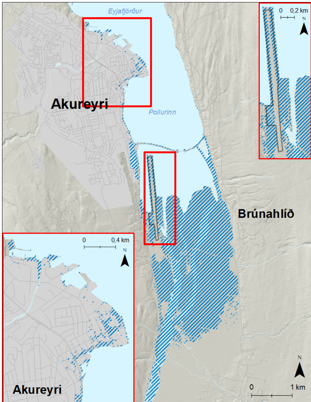
Mynd 126. Akureyri. Möguleg útbreiðsla sjávarflóðs sem hefur 50 ára endurkomutíma (2% árslíkur) við núverandi aðstæður.
