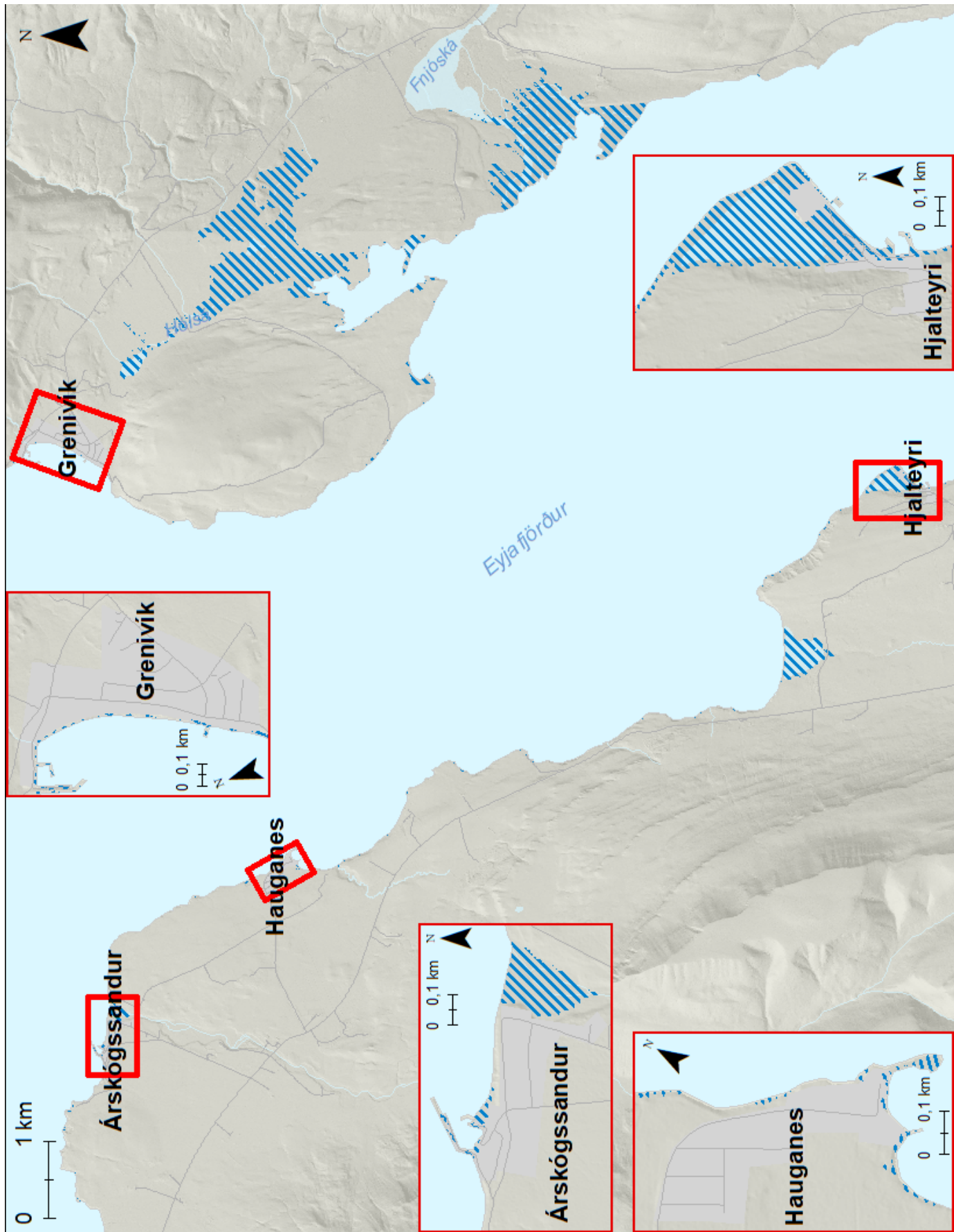
Mynd 65. Árskógssandur, Grenivík, Hauganes og Hjalteyri. Möguleg útbreiðsla sjávarflóðs sem hefur 20 ára endurkomutíma (5% árslíkur) árið 2150 miðað við sviðsmynd SSP5-8.5LC.
