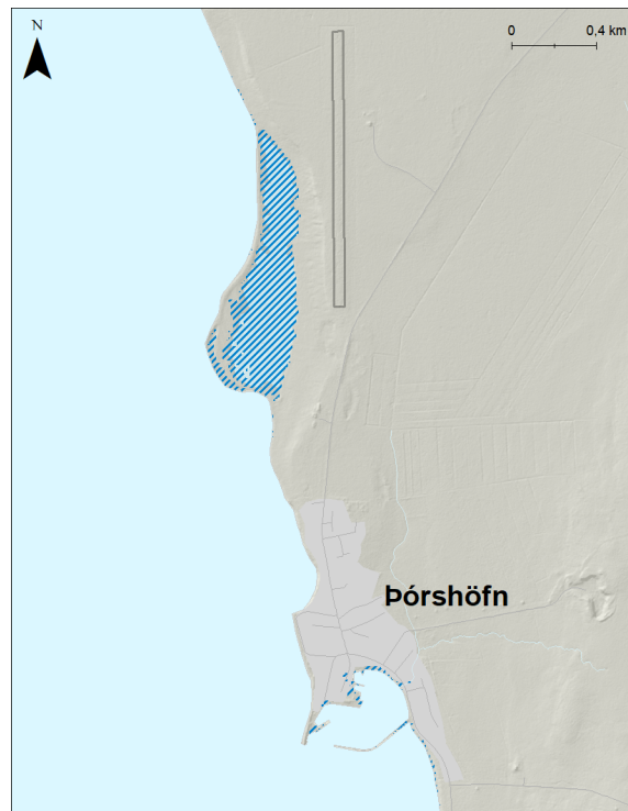
Mynd 250. Þórshöfn. Möguleg útbreiðsla sjávarflóðs sem hefur 50 ára endurkomutíma (2% árslíkur) árið 2100 miðað við sviðsmynd SSP5-8.5LC.
