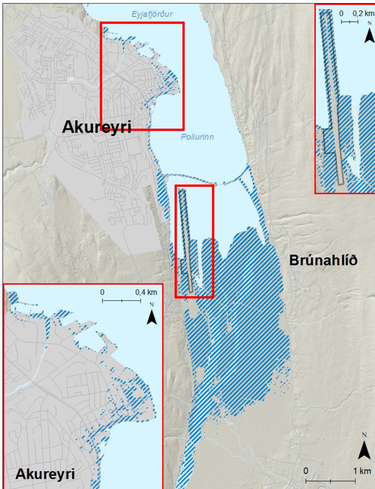
Mynd 124. Akureyri. Möguleg útbreiðsla sjávarflóðs sem hefur 20 ára endurkomutíma (5% árslíkur) árið 2150 miðað við sviðsmynd SSP5-8.5.
