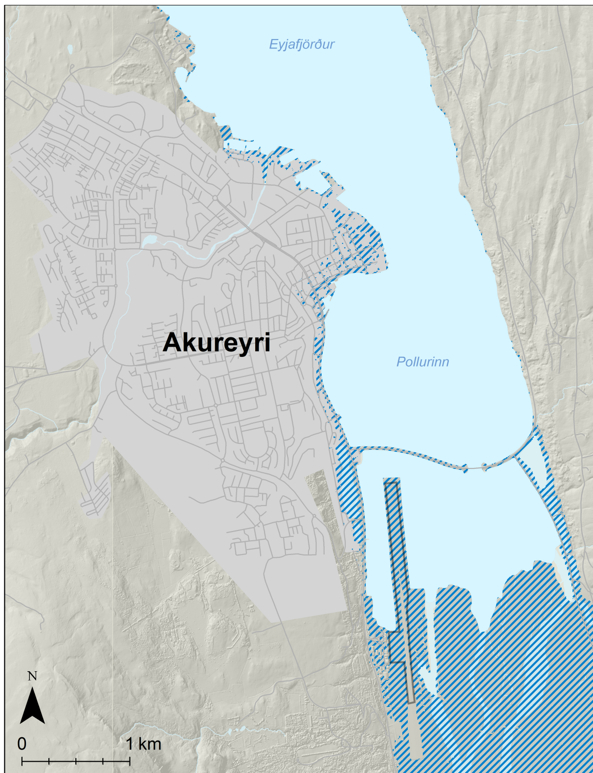
Mynd 148. Akureyri. Möguleg útbreiðsla sjávarflóðs sem hefur 200 ára endurkomutíma (0,5% árslíkur) árið 2100 miðað við sviðsmynd SSP5-8.5LC.
