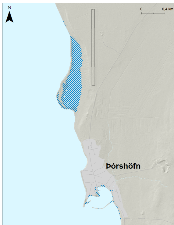
Mynd 253. Þórshöfn. Möguleg útbreiðsla sjávarflóðs sem hefur 200 ára endurkomutíma (0,5% árslíkur) árið 2150 miðað við sviðsmynd SSP5-8.5.
