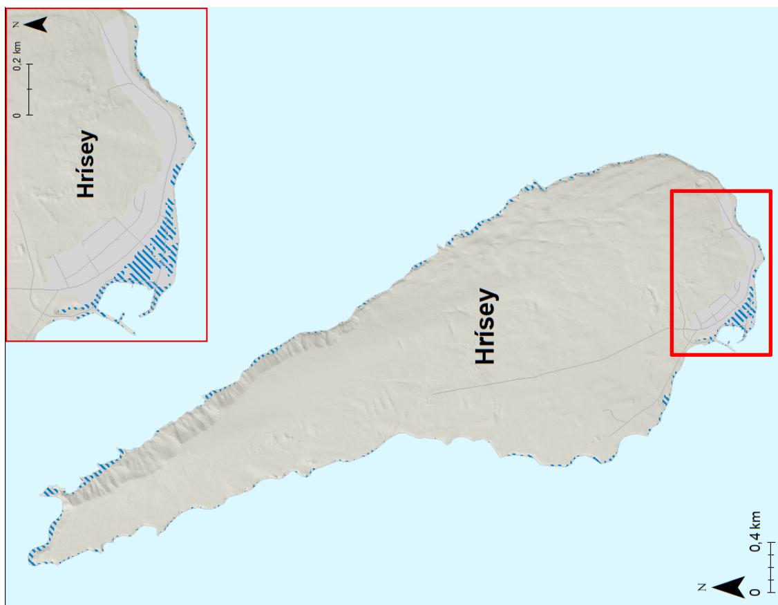
Mynd 52. Hrísey. Möguleg úbreiðsla sjávarflóðs sem hefur 20 ára endurkomutíma (0,5% árslíkur) árið 2150 miðað við sviðsmynd SSP5-8.5LC.
