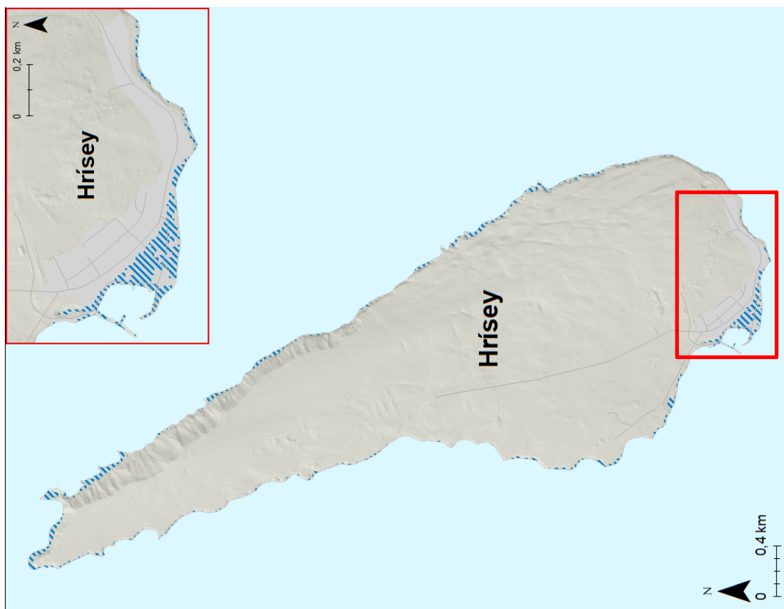
Mynd 60. Hrísey. Möguleg útbreiðsla sjávarflóðs sem hefur 200 ára endurkomutíma (0,5% árslíkur) árið 2150 miðað við sviðsmynd SSP5-8.5LC.
