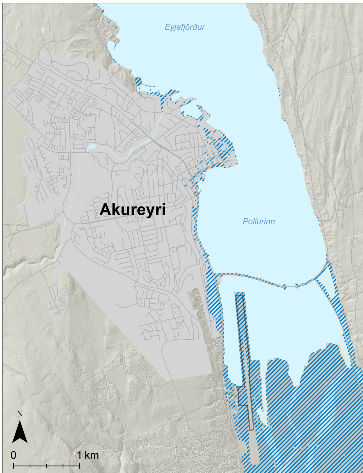
Mynd 143. Akureyri. Möguleg útbreiðsla sjávarflóðs sem hefur 50 ára endurkomutíma (2% árslíkur) árið 2100 miðað við sviðsmynd SSP5-8.5LC.
