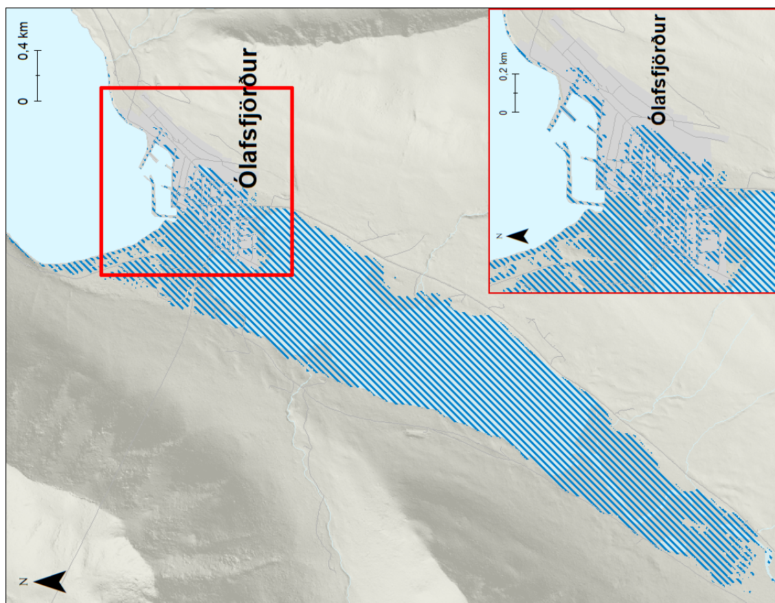
Mynd 25. Ólafsfjörður: Möguleg útbreiðsla sjávarflóðs sem hefur 50 ára endurkomutíma (0,5% árslíkur) árið 2100 miðað við sviðsmynd SSP5-8.5LC.
