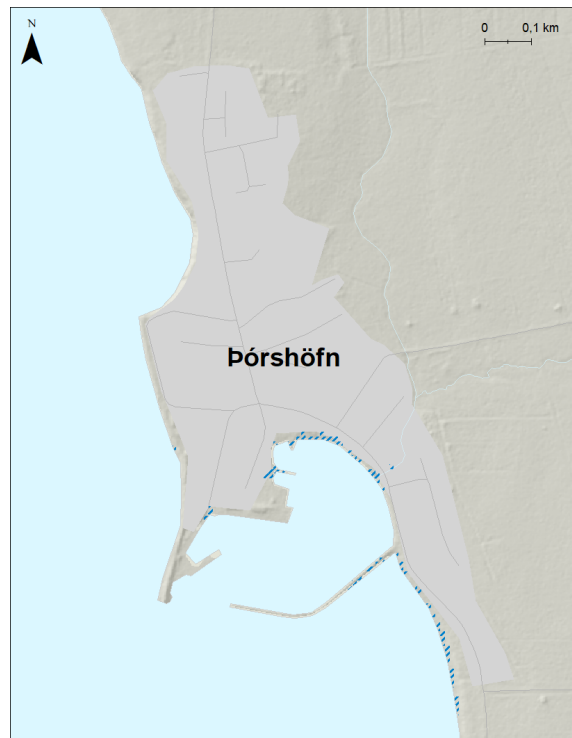
Mynd 258. Þórshöfn. Möguleg útbreiðsla sjávarflóðs sem hefur 200 ára endurkomutíma (0,5% árslíkur) við núverandi aðstæður.
