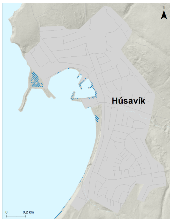
Mynd 208. Húsavík. Möguleg útbreiðsla sjávarflóðs sem hefur 200 ára endurkomutíma (0,5% árslíkur) árið 2150 miðað við sviðsmynd SSP5-8.5.
