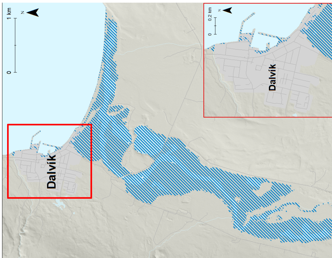
Mynd 37. Dalvík. Möguleg útbreiðsla sjávarflóðs sem hefur 50 ára endurkomutíma (0,5% árslíkur) árið 2100 miðað við sviðsmynd SSP5-8.5LC.
