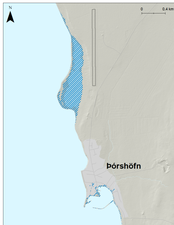
Mynd 255. Þórshöfn. Möguleg útbreiðsla sjávarflóðs sem hefur 200 ára endurkomutíma (0,5% árslíkur) árið 2150 miðað við sviðsmynd SSP5-8.5LC.
