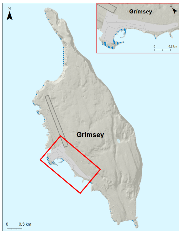
Mynd 185. Grímsey. Möguleg útbreiðsla sjávarflóðs sem hefur 20 ára endurkomutíma (5% árslíkur) árið 2150 miðað við sviðsmynd SSP5-8.5.
