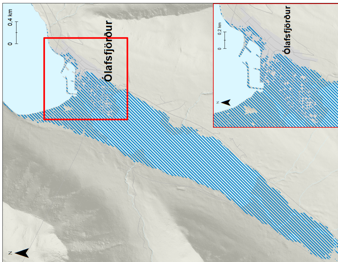
Mynd 30. Ólafsfjörður: Möguleg útbreiðsla sjávarflóðs sem hefur 200 ára endurkomutíma (0,5% árslíkur) árið 2150 miðað við sviðsmynd SSP5-8.5LC.
