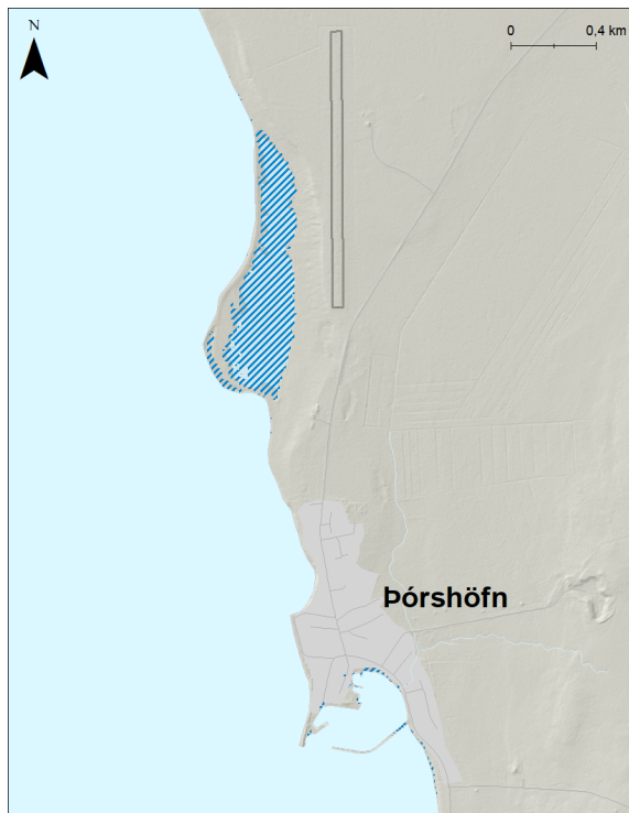
Mynd 244. Þórshöfn. Möguleg útbreiðsla sjávarflóðs sem hefur 20 ára endurkomutíma (5% árslíkur) árið 2100 miðað við sviðsmynd SSP5-8.5.
