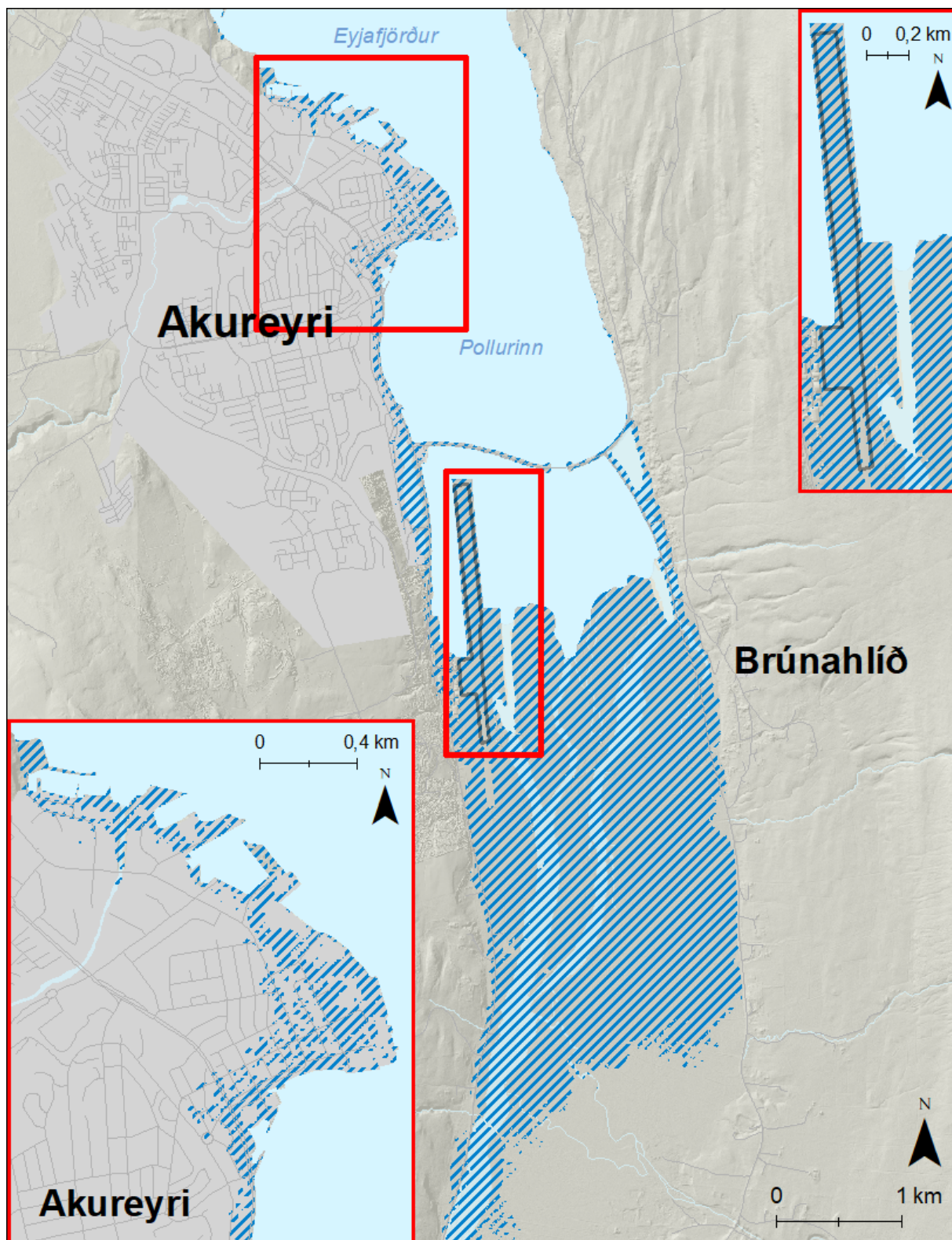
Mynd 135. Akureyri. Möguleg útbreiðsla sjávarflóðs sem hefur 200 ára endurkomutíma (0,5% árslíkur) árið 2150 miðað við sviðsmynd SSP5-8.5LC.
