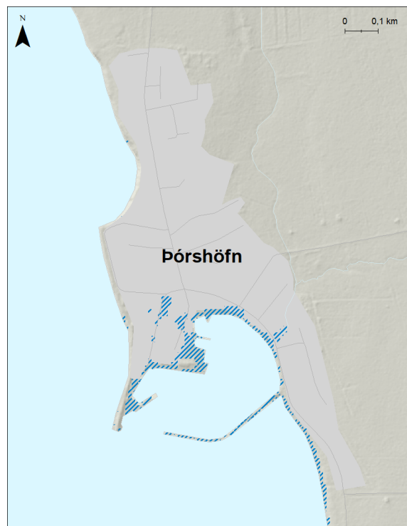
Mynd 270. Þórshöfn. Möguleg útbreiðsla sjávarflóðs sem hefur 200 ára endurkomutíma (0,5% árslíkur) árið 2150 miðað við sviðsmynd SSP5-8.5LC.
