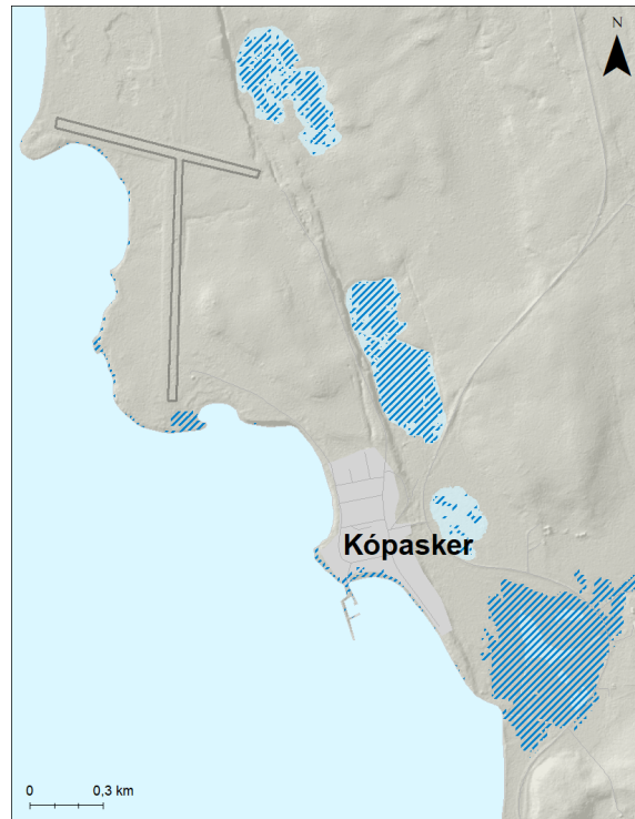
Mynd 224. Kópasker. Möguleg útbreiðsla sjávarflóðs sem hefur 200 ára endurkomutíma (0,5% árslíkur) árið 2100 miðað við sviðsmynd SSP5-8.5LC.
