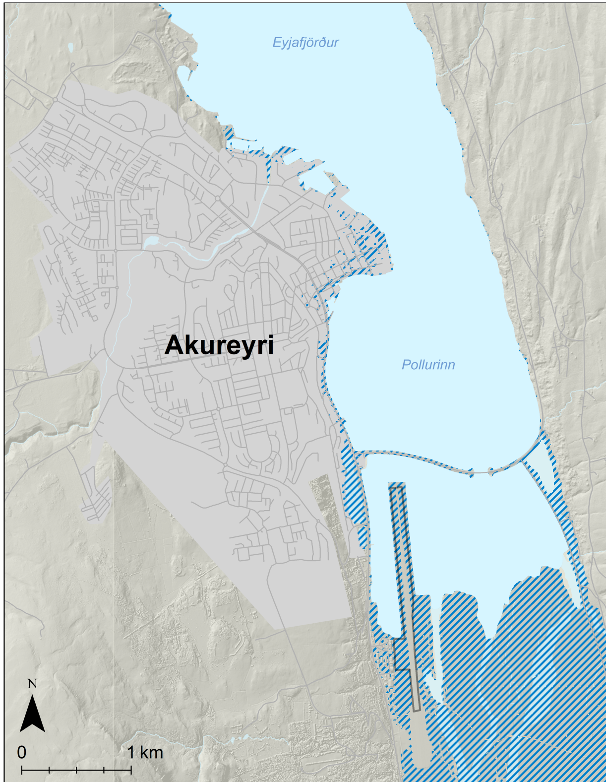
Mynd 146. Akureyri. Möguleg útbreiðsla sjávarflóðs sem hefur 200 ára endurkomutíma (0,5% árslíkur) við núverandi aðstæður.
