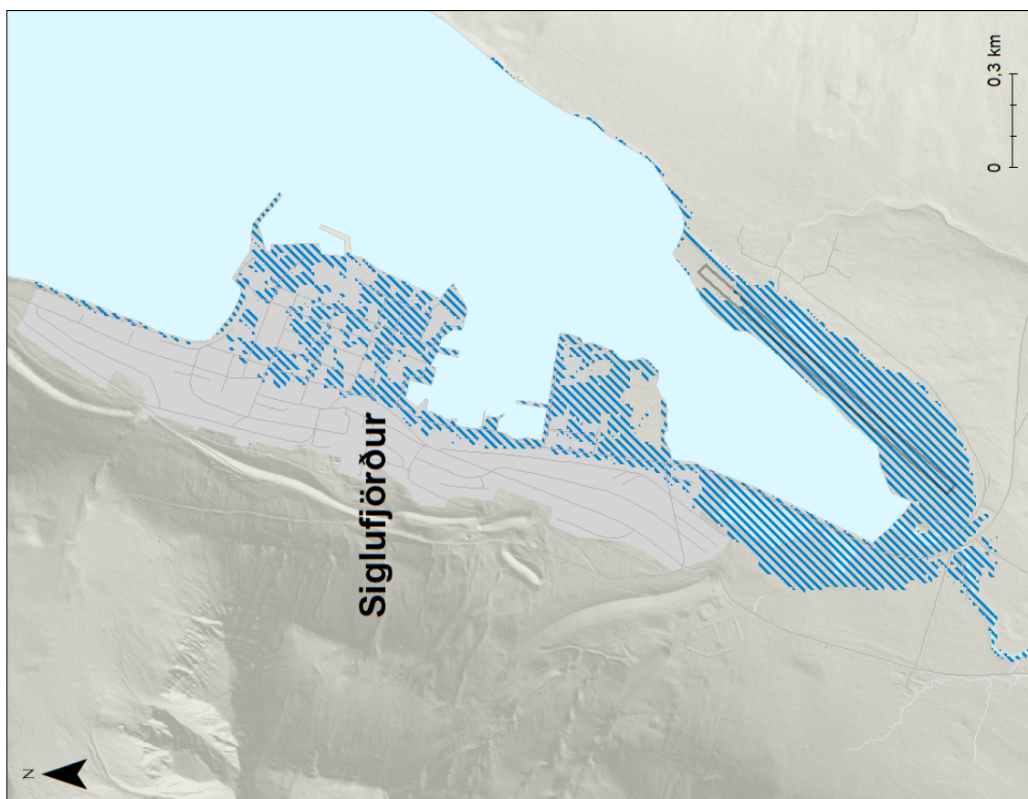
Mynd 7. Siglufjörður. Möguleg útbreiðsla sjávarflóðs sem hefur 50 ára endurkomutíma (0,5% árslíkur) árið 2100 miðað við sviðsmynd SSP5-8.5LC.
