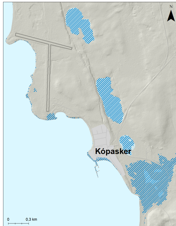
Mynd 225. Kópasker. Möguleg útbreiðsla sjávarflóðs sem hefur 200 ára endurkomutíma (0,5% árslíkur) árið 2150 miðað við sviðsmynd SSP5-8.5LC.
