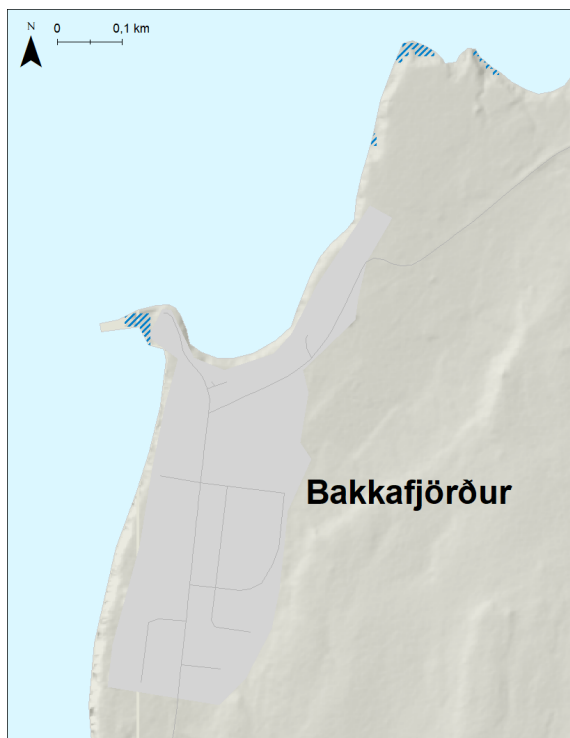
Mynd 272. Bakkafljóðs. Möguleg útbreiðsla sjávarflóðs sem hefur 50 ára endurkomutíma (2% árslíkur) við núverandi aðstæður.
