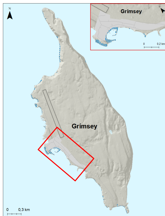
Mynd 191. Grímsey. Möguleg útbreiðsla sjávarflóðs sem hefur 50 ára endurkomutíma (2% árslíkur) árið 2150 miðað við sviðsmynd SSP5-8.5LC.
