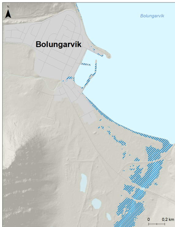
Mynd 121. Bolungarvík. Möguleg útbreiðsla sjávarflóðs sem hefur 20 ára endurkomutíma (5% árslíkur) við núverandi aðstæður.
