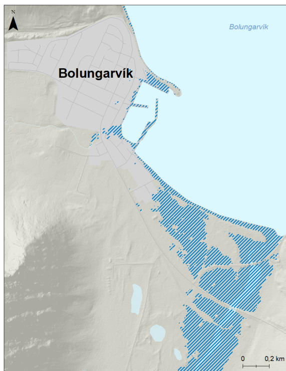
Mynd 133. Bolungarvík. Möguleg útbreiðsla sjávarflóðs sem hefur 200 ára endurkomutíma (0,5% árslíkur) árið 2150 miðað við sviðsmynd SSP5-8.5.
