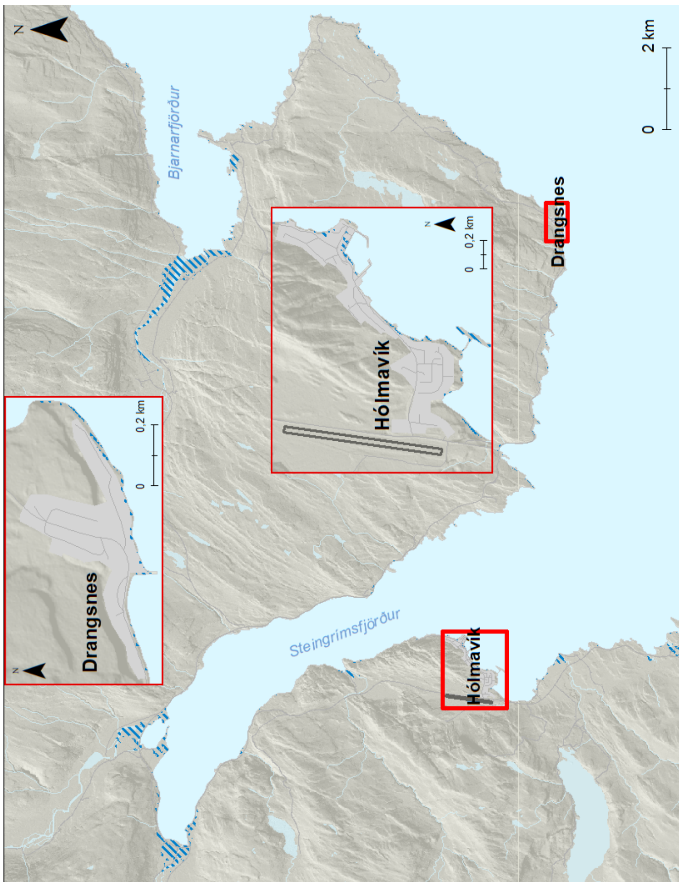
Mynd 181. Drangsnæs og Hólmavík. Möguleg útbreiðsla sjávarflóðs sem hefur 20 ára endurkomutíma (5% árslíkur) við núverandi aðstæður.
