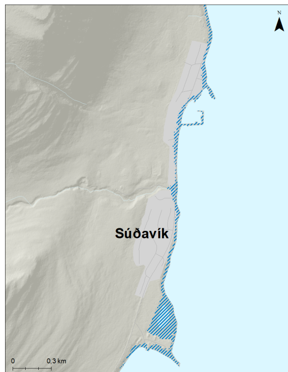
Mynd 180. Súðavík. Möguleg útbreiðsla sjávarflóðs sem hefur 200 ára endurkomutíma (0,5% árslíkur) árið 2150 miðað við sviðsmynd SSP5-8.5LC.
