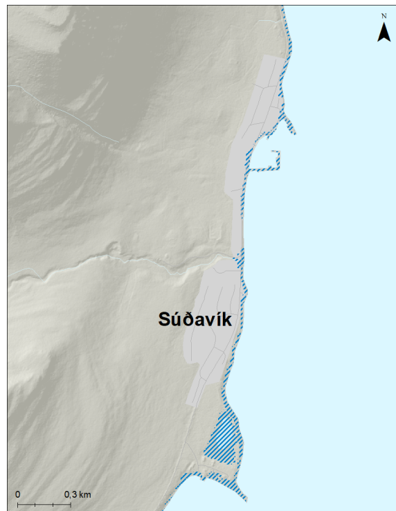
Mynd 175. Súðavík. Möguleg útbreiðsla sjávarflóðs sem hefur 50 ára endurkomutíma (2% árslíkur) árið 2100 miðað við sviðsmynd SSP5-8.5LC.
