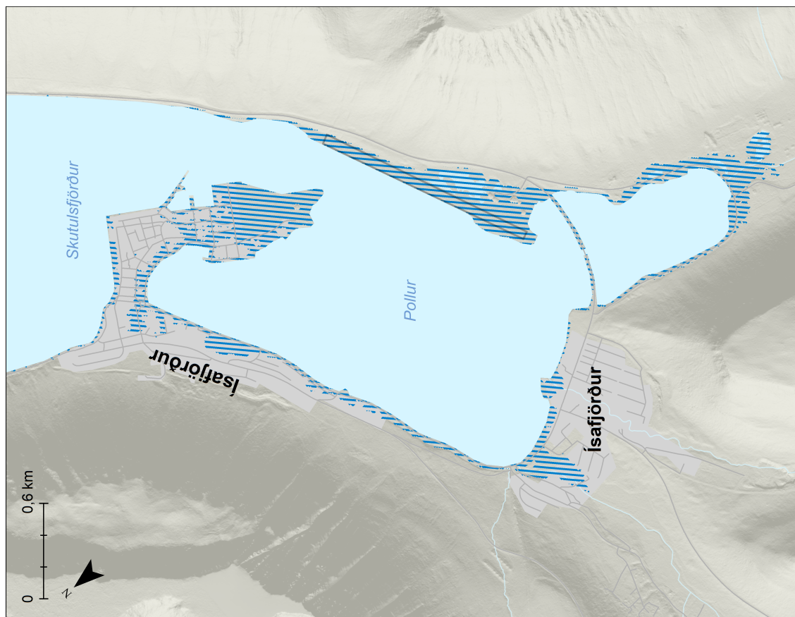
Mynd 153. Ísafjörður. Möguleg útbreiðsla sjávarflóðs sem hefur 200 ára endurkomutíma (0,5% árslíkur) við núverandi aðstæður.
