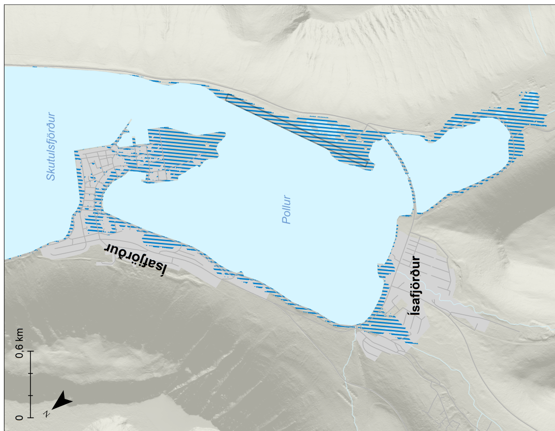
Mynd 160. Ísafjörður. Möguleg útbreiðsla sjávarflóðs sem hefur 50 ára endurkomutíma (0,5% árslíkur) árið 2100 miðað við sviðsmynd SSP5-8.5LC.
