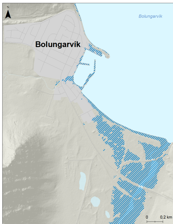
Mynd 129. Bolungarvík. Möguleg útbreiðsla sjávarflóðs sem hefur 50 ára endurkomutíma (2% árslíkur) árið 2150 miðað við sviðsmynd SSP5-8.5.
