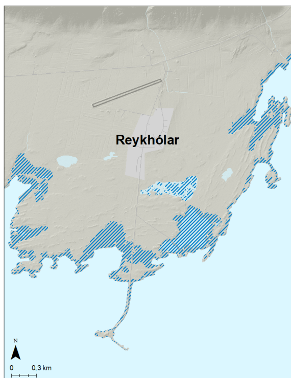
Mynd 2. Reykhólar. Möguleg útbreiðsla sjávarflóðs sem hefur 50 ára endurkomutíma (2% árslíkur) við núverandi aðstæður.
