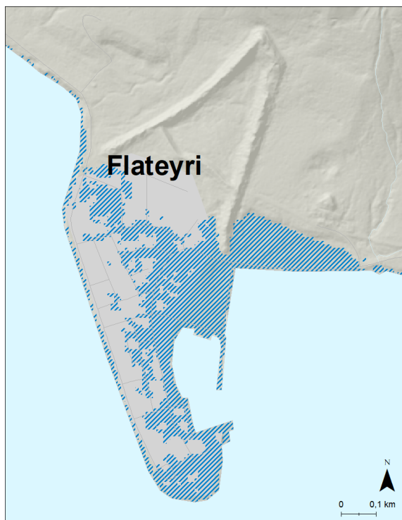
Mynd 99. Flateyri. Möguleg útbreiðsla sjávarflóðs sem hefur 50 ára endurkomutíma (2% árslíkur) árið 2150 miðað við sviðsmynd SSP5-8.5.
