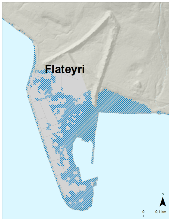
Mynd 102. Flateyri. Möguleg útbreiðsla sjávarflóðs sem hefur 200 ára endurkomutíma (0,5% árslíkur) árið 2100 miðað við sviðsmynd SSP5-8.5.
