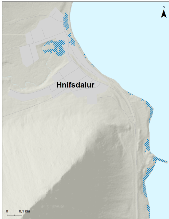
Mynd 143. Hnífsdalur. Möguleg útbreiðsla sjávarflóðs sem hefur 50 ára endurkomutíma (2% árslíkur) árið 2100 miðað við sviðsmynd SSP5-8.5.
