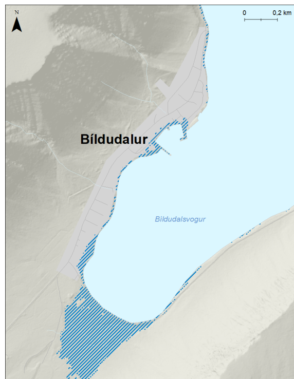
Mynd 75. Bíldudalur. Möguleg útbreiðsla sjávarflóðs sem hefur 200 ára endurkomutíma (0,5% árslíkur) árið 2150 miðað við sviðsmynd SSP5-8.5LC.
