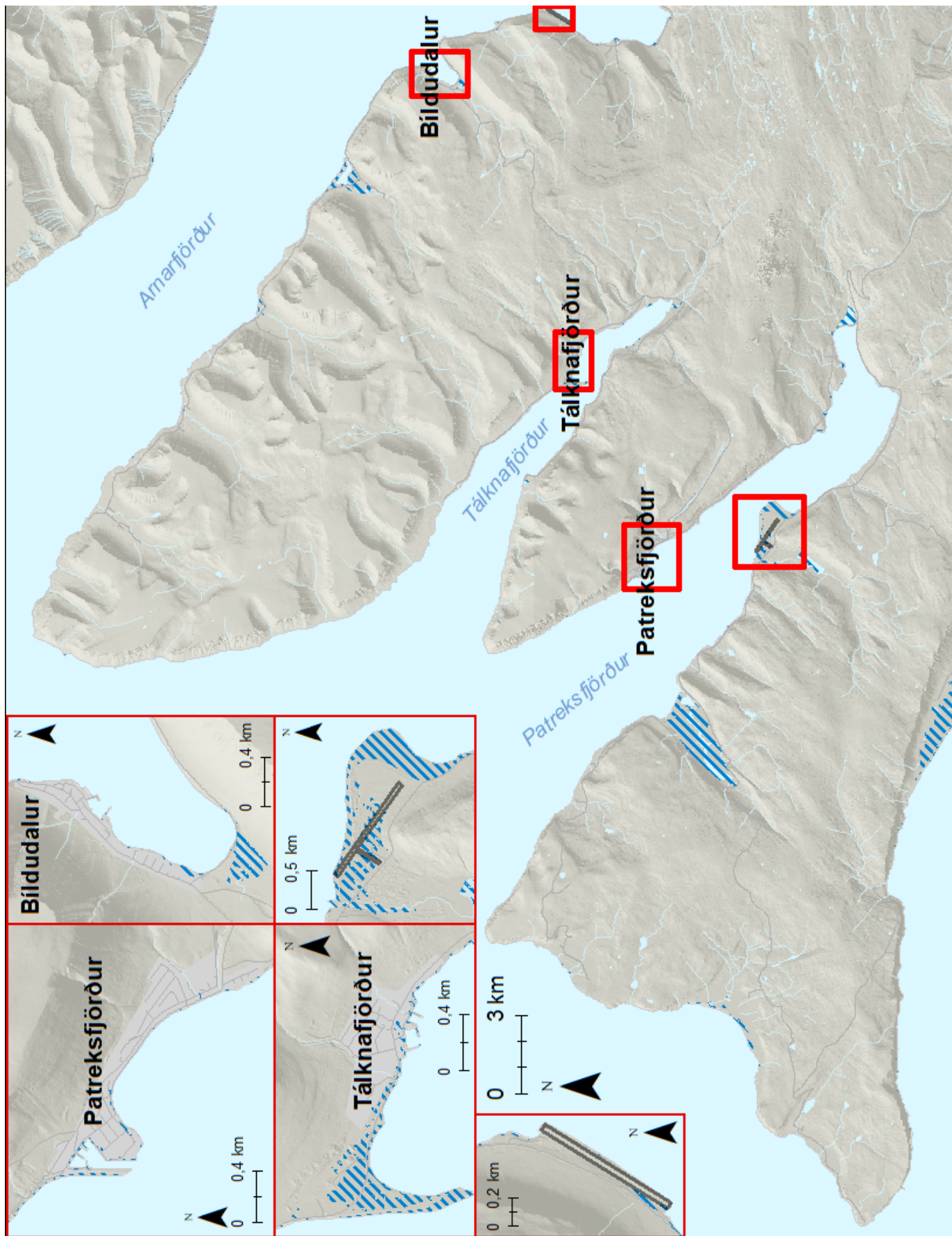
Mynd 16. Patreksfjörður, Tálknafjörður og Bildudalur. Möguleg útbreiðsla sjávarflóðs sem hefur 20 ára endurkomutíma (5% árslíkur) við núverandi aðstæður.
