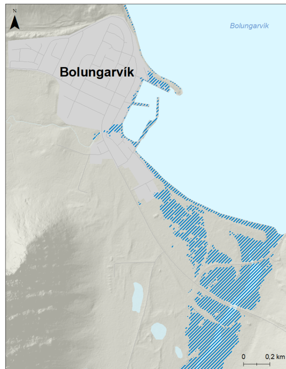
Mynd 130. Bolungarvík. Möguleg útbreiðsla sjávarflóðs sem hefur 50 ára endurkomutíma (2% árslíkur) árið 2100 miðað við sviðsmynd SSP5-8.5LC.
