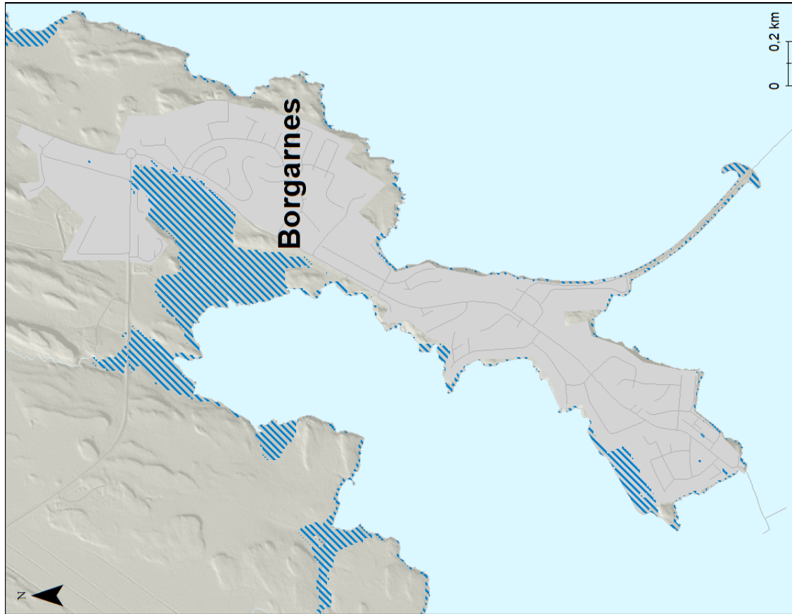
Mynd 60. Borgarnes. Möguleg útbreiðsla sjávarflóðs sem hefur 200 ára endurkomutíma (0,5% árslíkur) við núverandi aðstæður.
