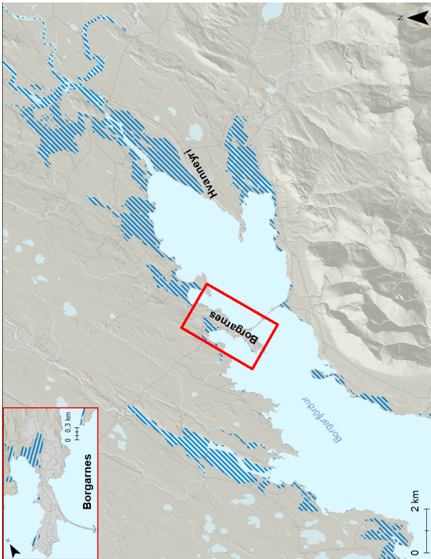
Mynd 17. Borgarfjörður. Möguleg útbreiðsla sjávarflóðs sem hefur 20 ára endurkomutíma (5% árslíkur) árið 2100 miðað við sviðsmynd SSP5-8.5.
