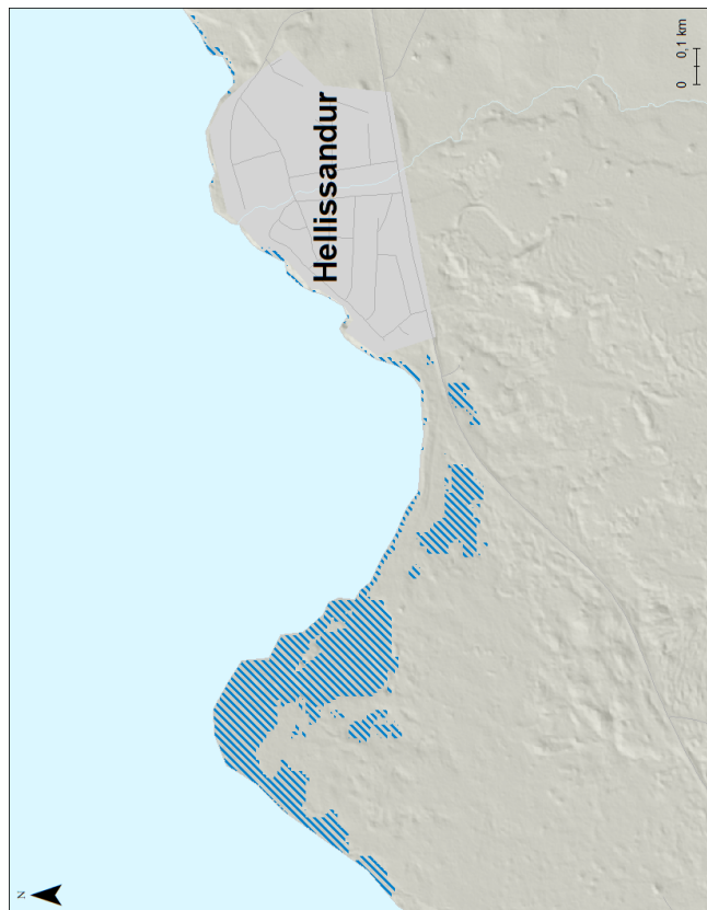
Mynd 93. Hellissandur. Möguleg útbreiðsla sjávarflóðs sem hefur 200 ára endurkomutíma (0,5% árslíkur) við núverandi aðstæður.
