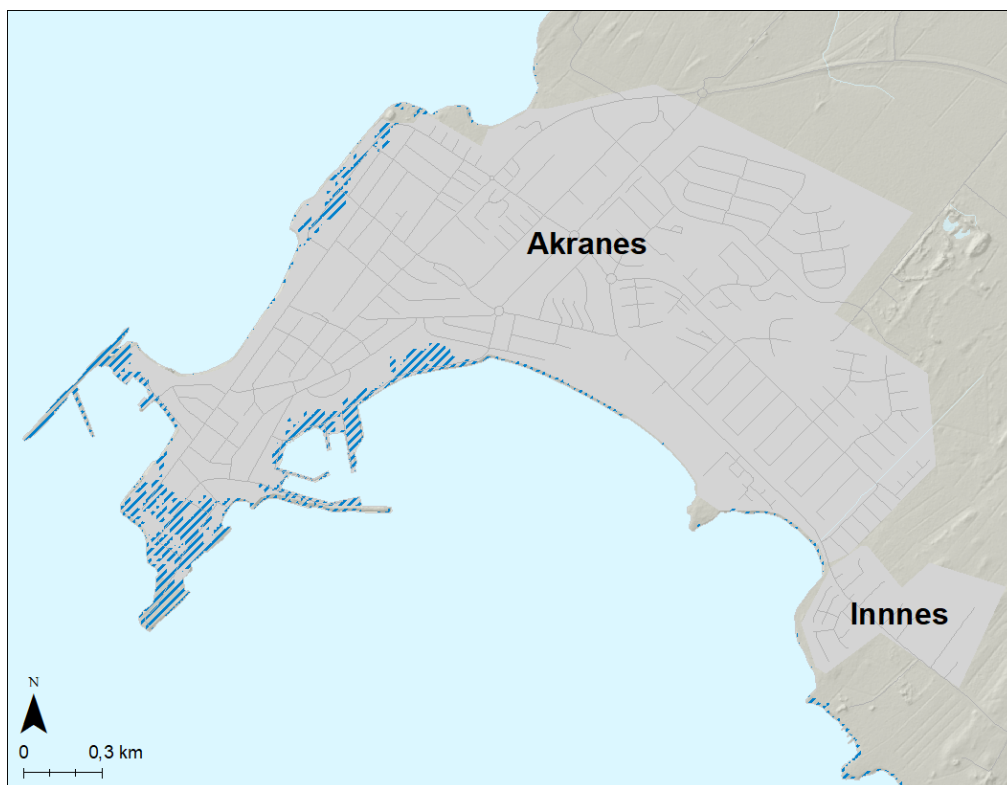
Mynd 15. Akranes. Möguleg útbreiðsla sjávarflóðs sem hefur 200 ára endurkomutíma (0,5% árslíkur) árið 2150 miðað við sviðsmynd SSP5-8.5LC.
