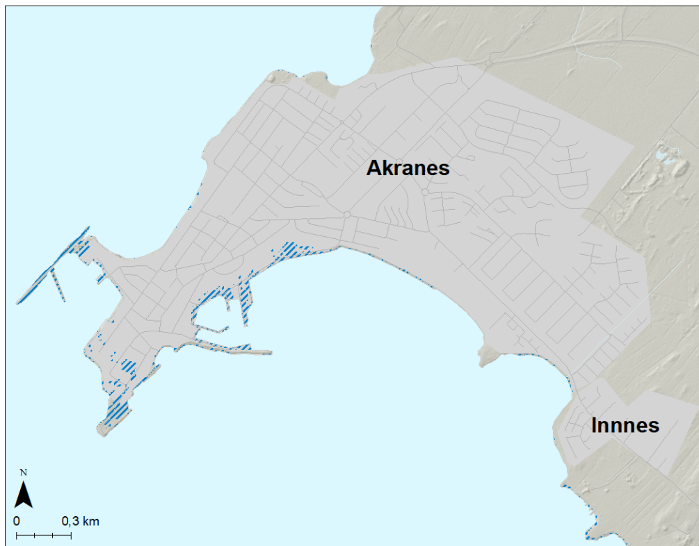
Mynd 4. Akranes. Möguleg útbreiðsla sjávarflóðs sem hefur 20 ára endurkomutíma (0,5% árslíkur) árið 2100 miðað við sviðsmynd SSP5-8.5.
