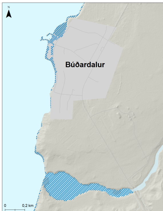
Mynd 189. Búðardalur. Möguleg útbreiðsla sjávarflóðs sem hefur 50 ára endurkomutíma (2% árslíkur) árið 2150 miðað við sviðsmynd SSP5-8.5.
