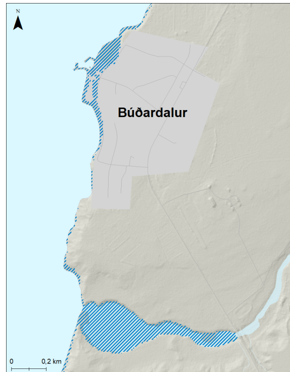
Mynd 195. Búðardalur. Möguleg útbreiðsla sjávarflóðs sem hefur 200 ára endurkomutíma (0,5% árslíkur) árið 2150 miðað við sviðsmynd SSP5-8.5LC.
