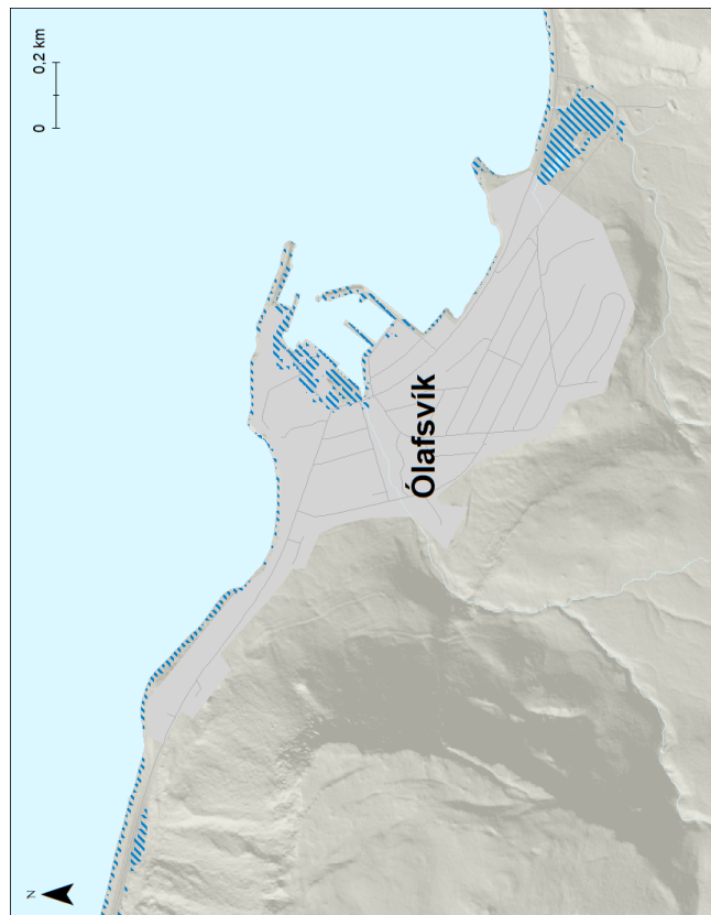
Mynd 123. Ólafsvík. Möguleg útbreiðsla sjávarflóðs sem hefur 200 ára endurkomutíma (0,5% árslíkur) við núverandi aðstæður.
