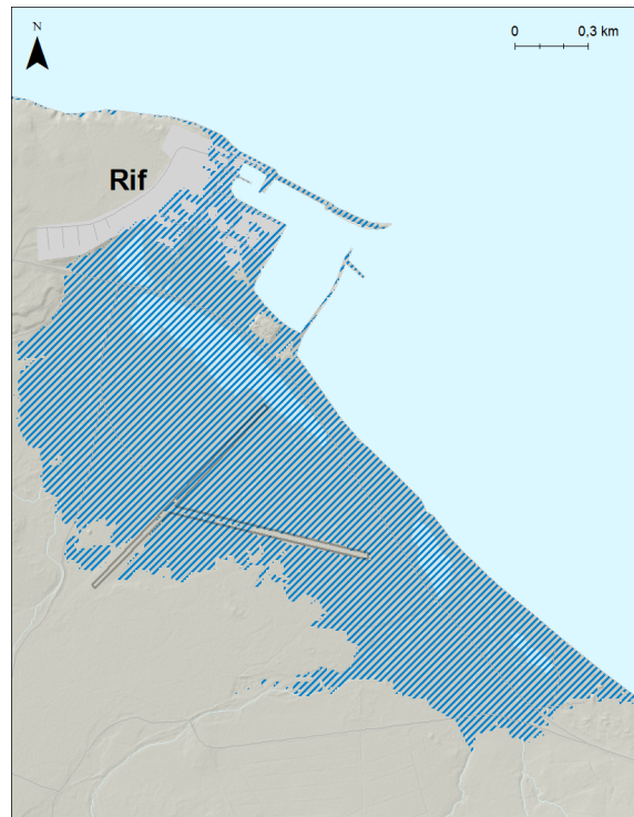
Mynd 116. Rif. Möguleg útbreiðsla sjávarflóðs sem hefur 50 ára endurkomutíma (2% árslíkur) árið 2150 miðað við sviðsmynd SSP5-8.5LC.
