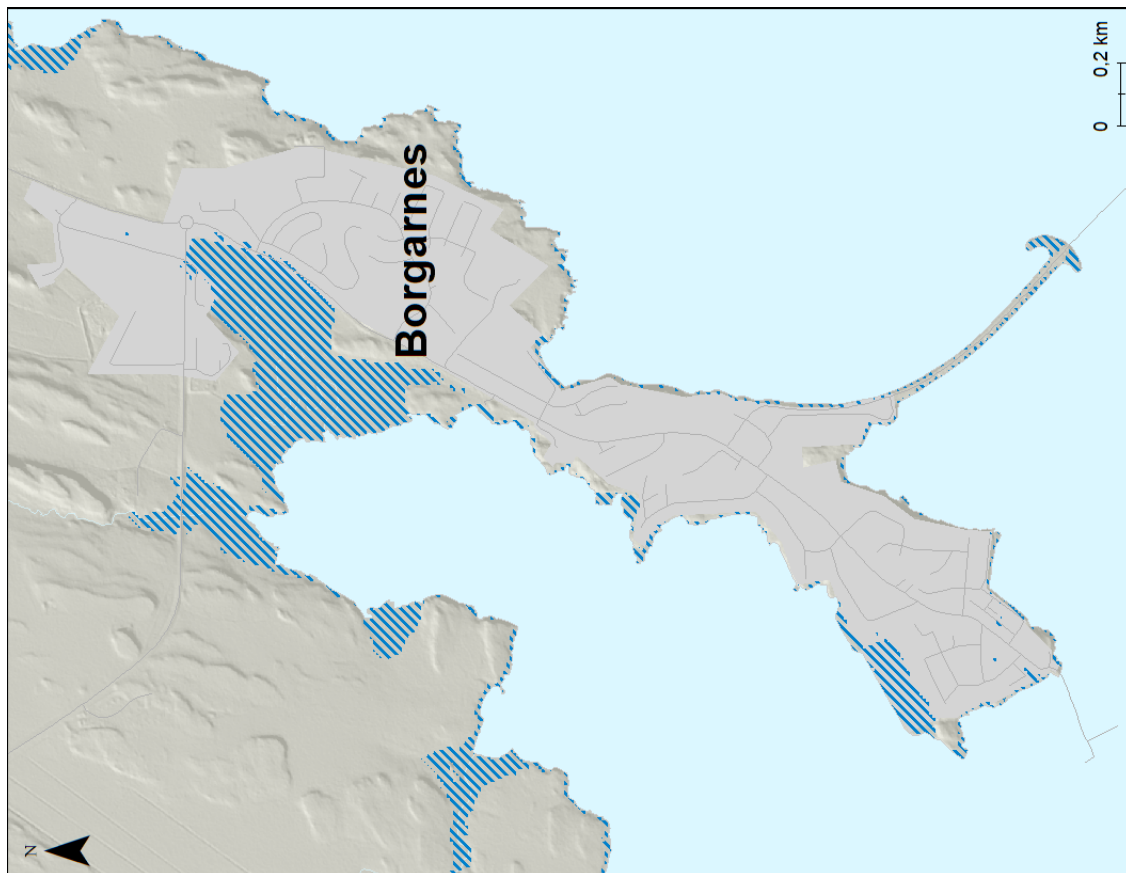
Mynd 50. Borgarnes. Möguleg útbreiðsla sjávarflóðs sem hefur 50 ára endurkomutíma (0,5% árslíkur) árið 2100 miðað við sviðsmynd SSP5-8.5.
