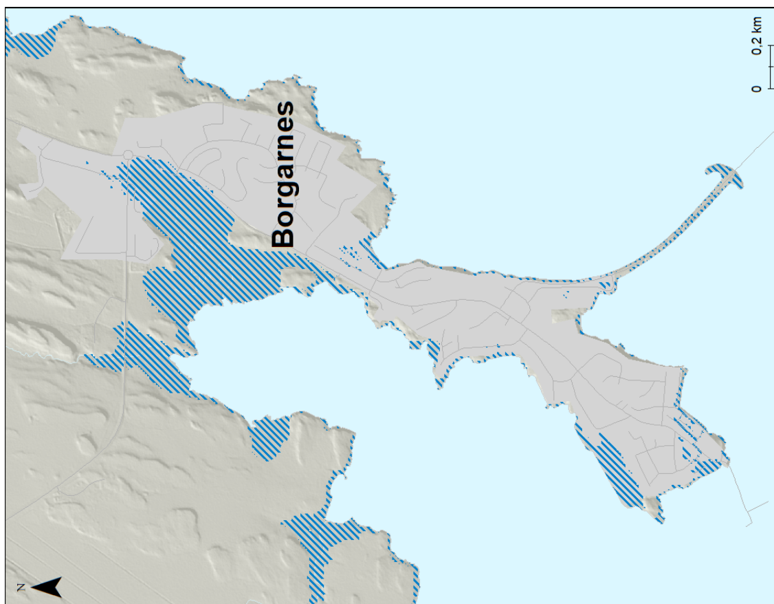
Mynd 57. Borgarnes. Möguleg útbreiðsla sjávarflóðs sem hefur 200 ára endurkomutíma (0,5% árslíkur) árið 2150 miðað við sviðsmynd SSP5-8.5LC.
