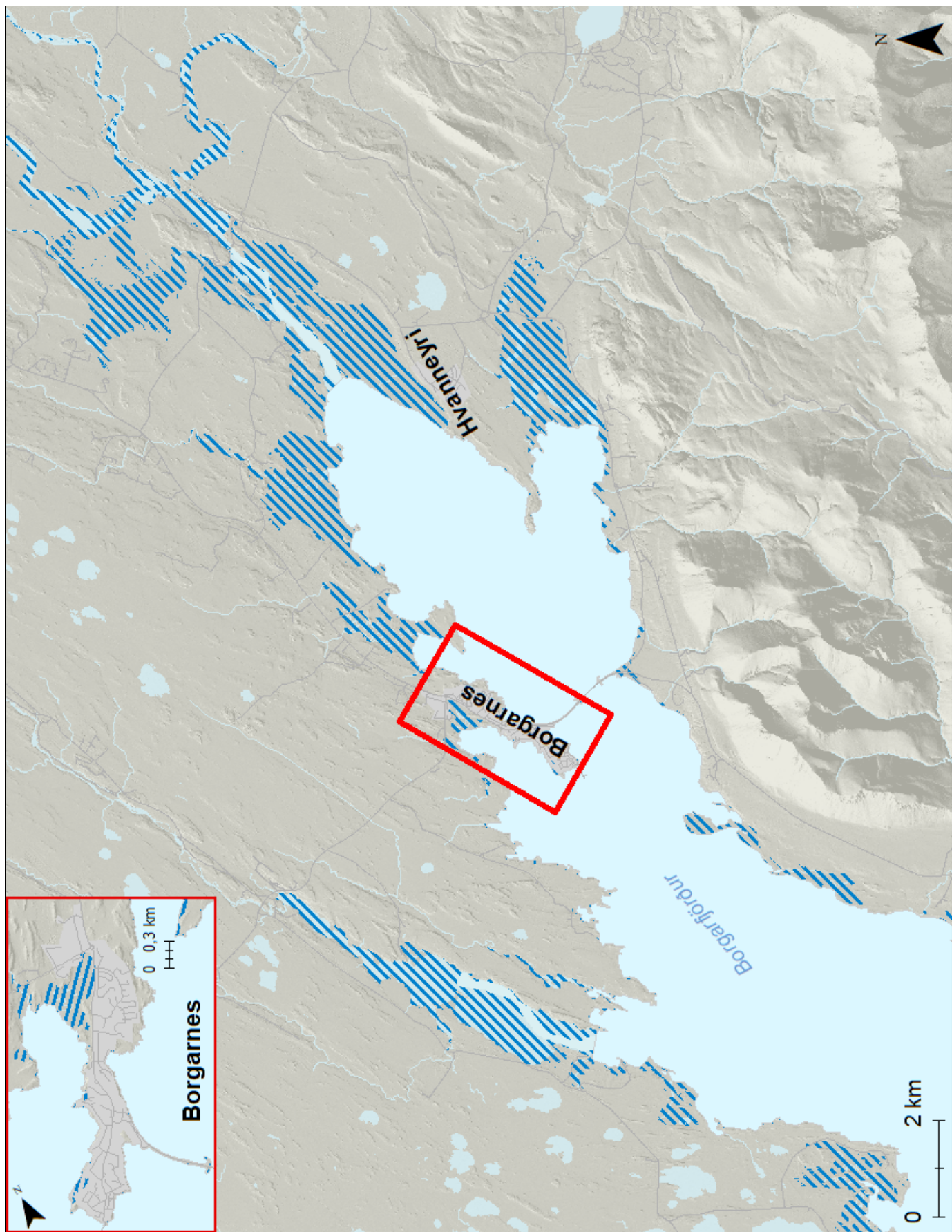
Mynd 21. Borgarfjörður. Möguleg útbreiðsla sjávarflóðs sem hefur 50 ára endurkomutíma (2% árslíkur) við núverandi aðstæður.
