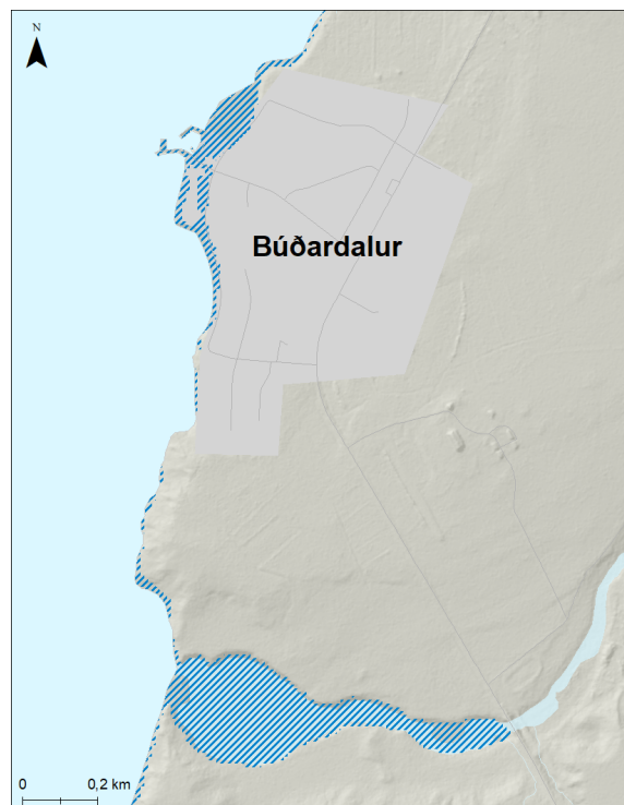
Mynd 191. Búðardalur. Möguleg útbreiðsla sjávarflóðs sem hefur 50 ára endurkomutíma (2% árslíkur) árið 2150 miðað við sviðsmynd SSP5-8.5LC.
