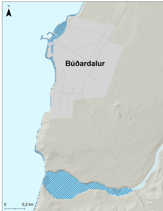
Mynd 184. Búðardalur. Möguleg útbreiðsla sjávarflóðs sem hefur 20 ára endurkomutíma (5% árslíkur) árið 2100 miðað við sviðsmynd SSP5-8.5.
