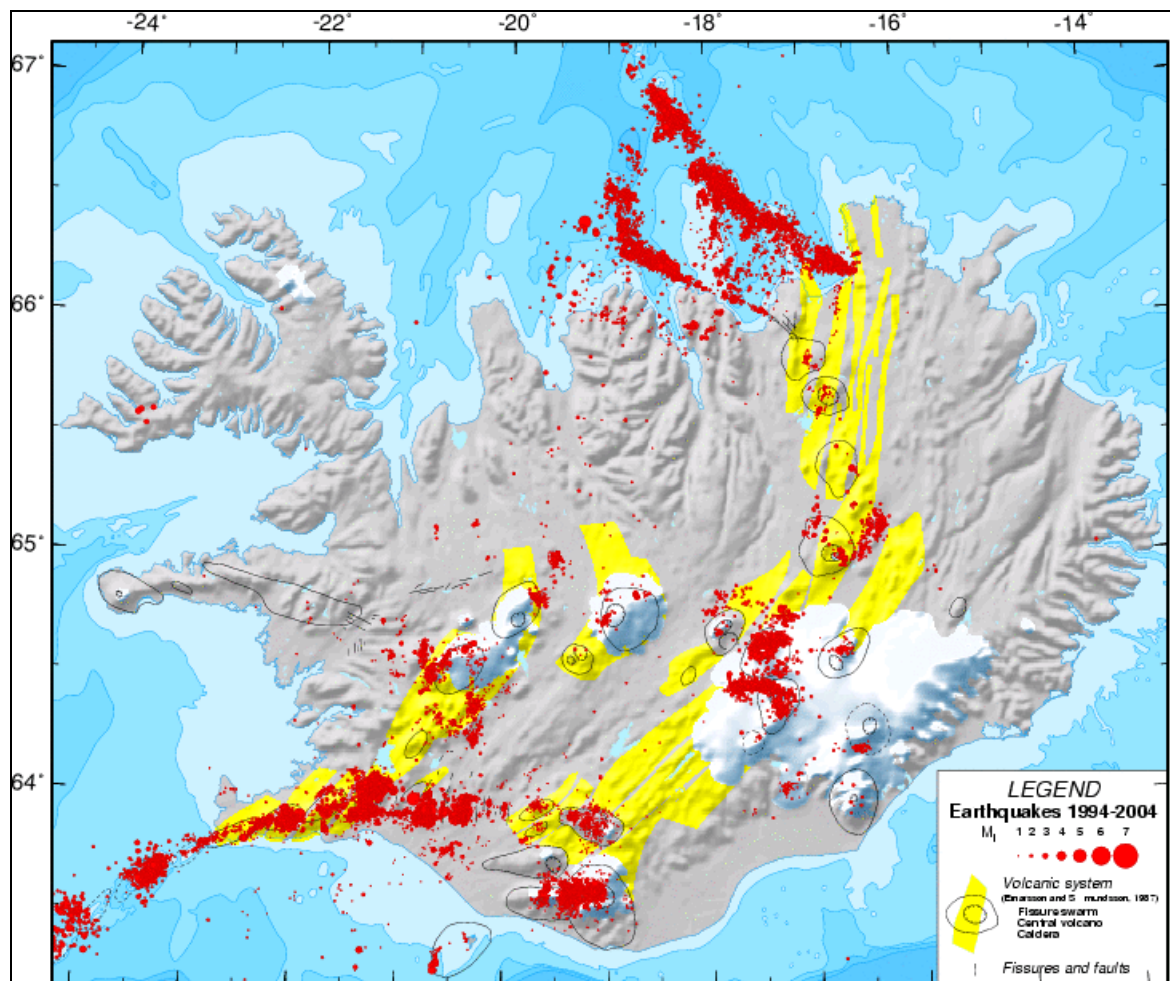
Mynd 1-1. Jarðskjálftavirkni á Íslandi 1994 til 2004. Myndin sýnir einnig eldvirku svæðin og megineldstöðvar (Gunnar B. Guðmundsson 2005).
